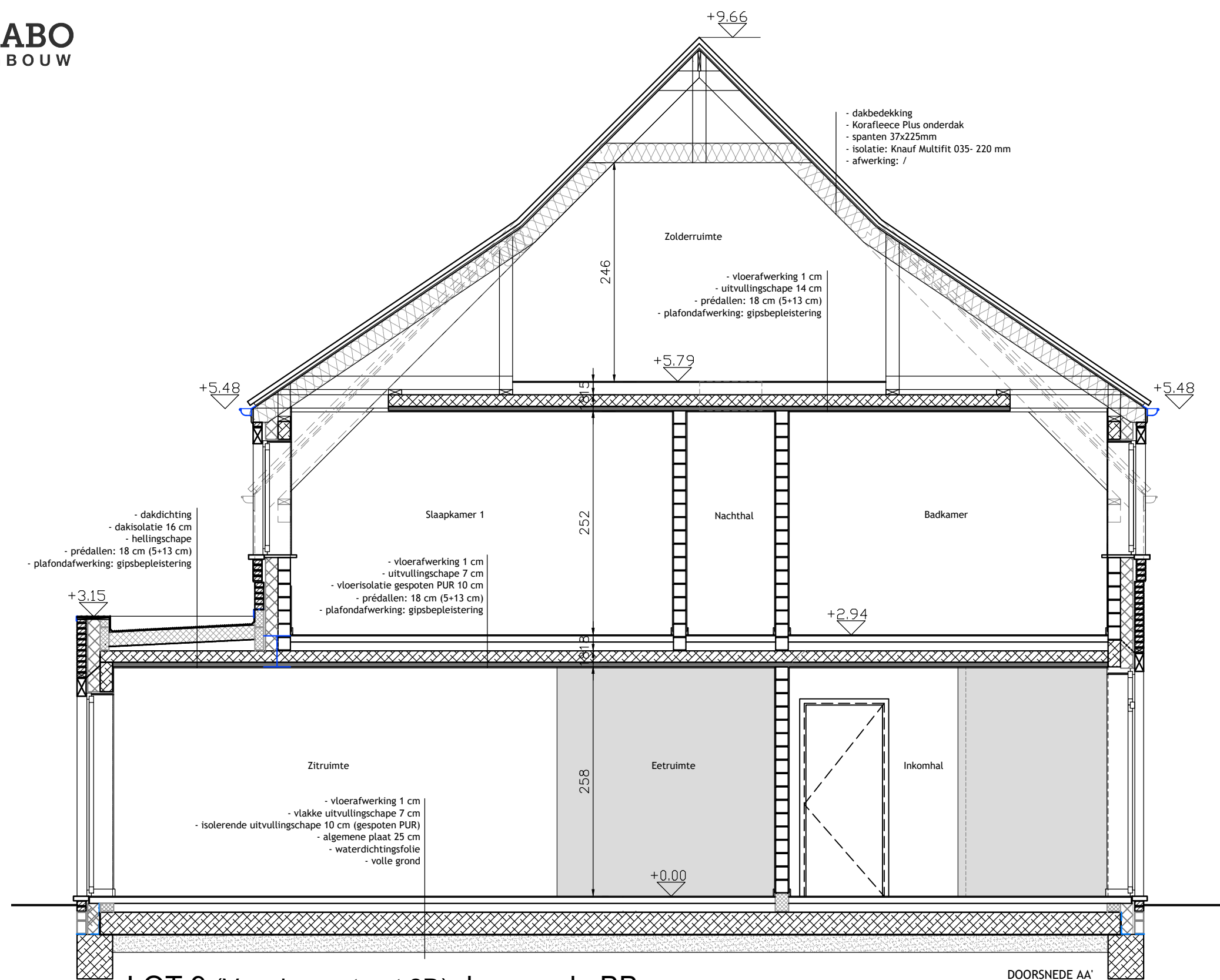
LOT 9 (Vogelzangstraat 2D) doorsnede BB schaal 1/50
