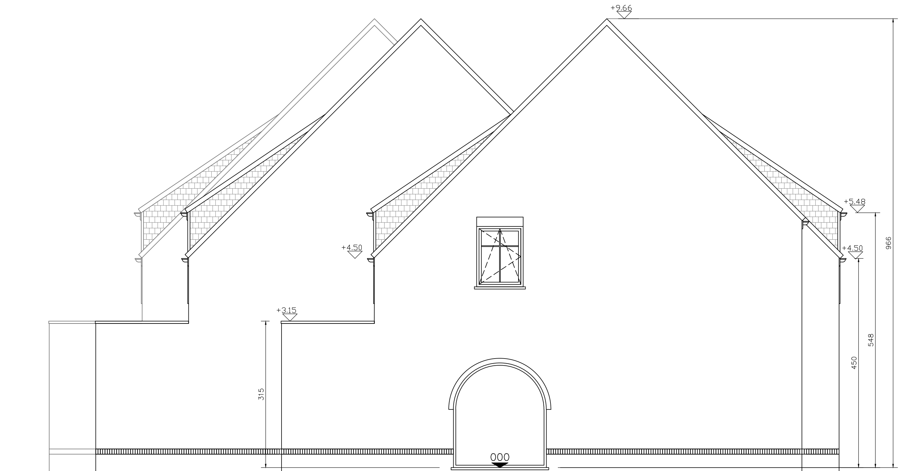
LOT 8 (Vogelzangstraat 2C) zijgevel links schaal 1/50
