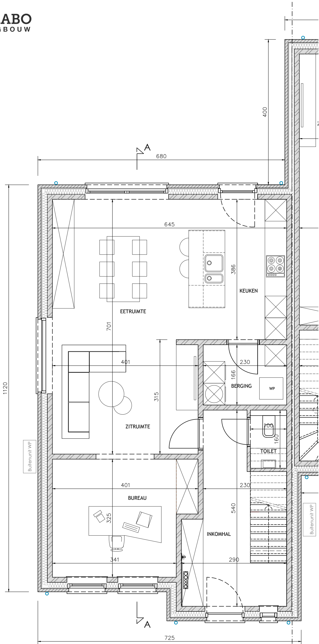
LOT 8 (Vogelzangstraat 2C) gelijkvloers schaal 1/50
