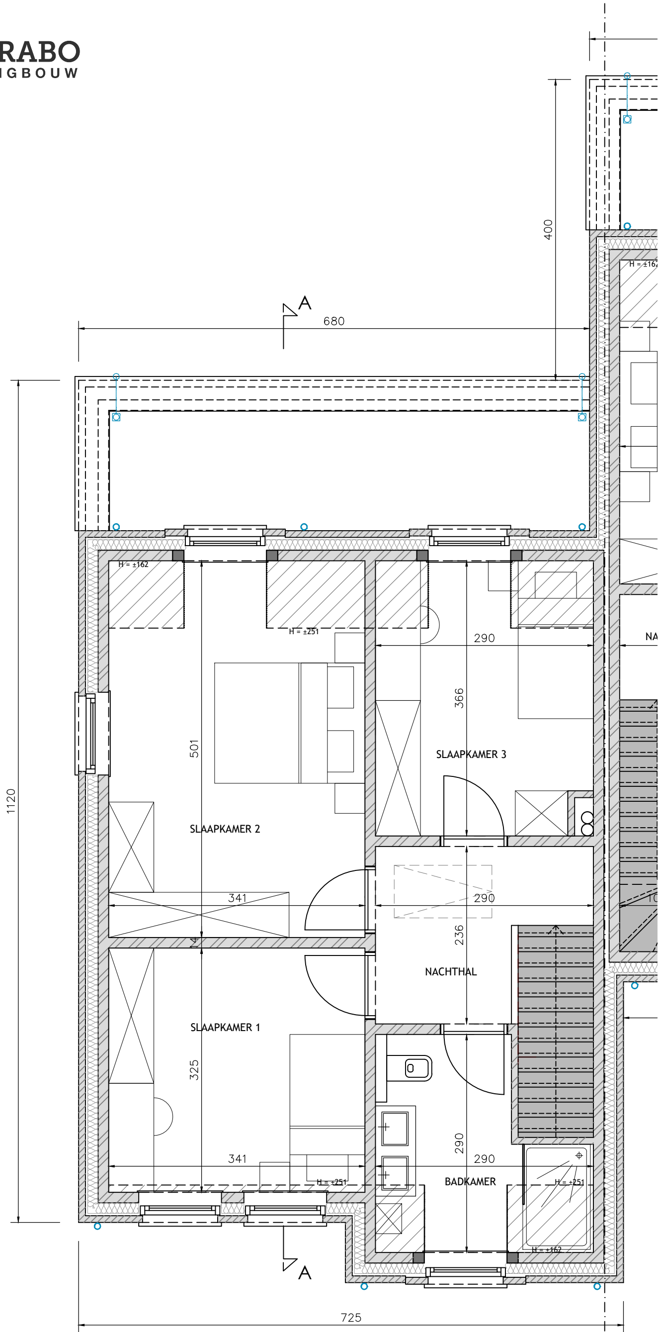
LOT 8 (Vogelzangstraat 2C) verdieping schaal 1/50
