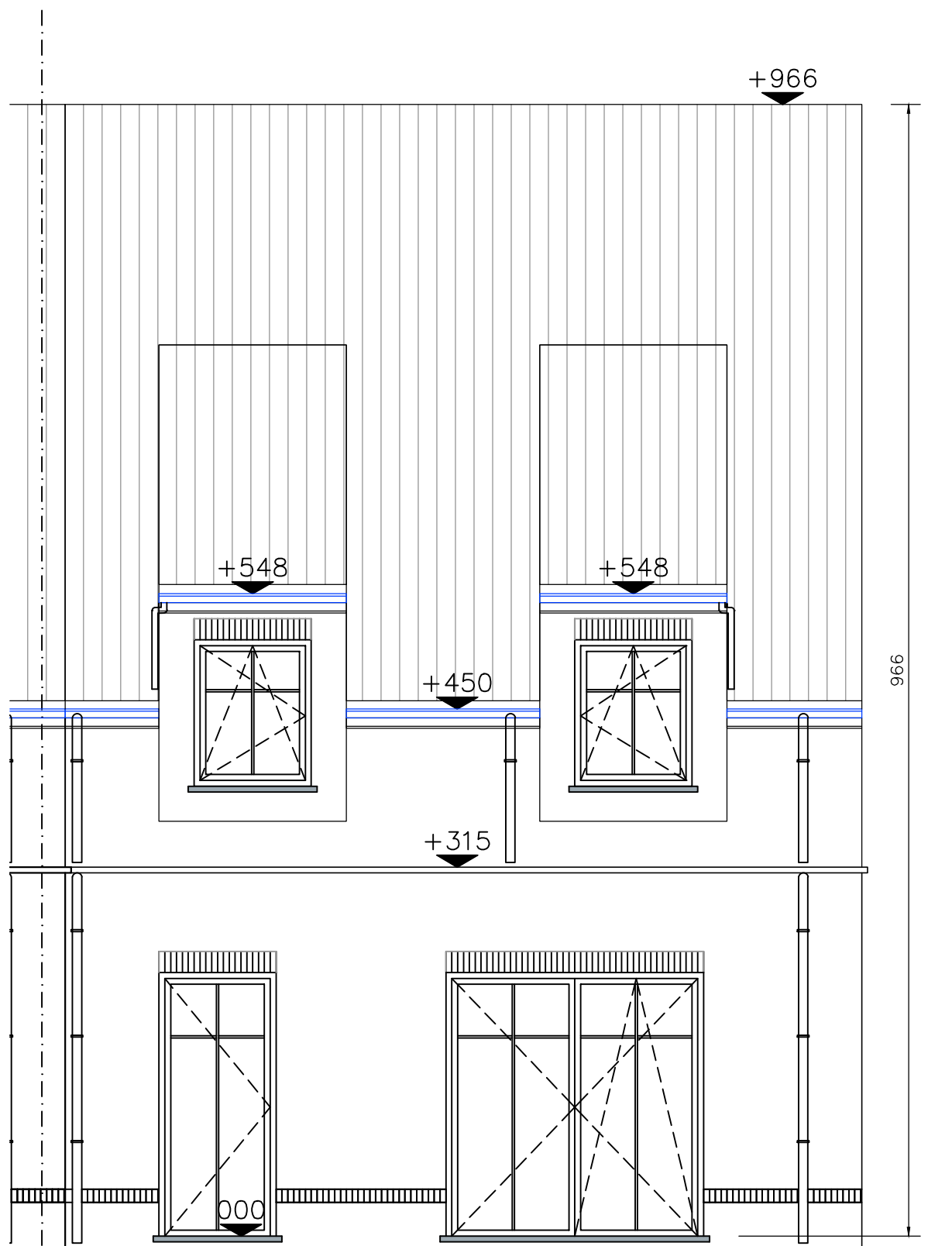
LOT 8 (Vogelzangstraat 2C) achtergevel schaal 1/50
