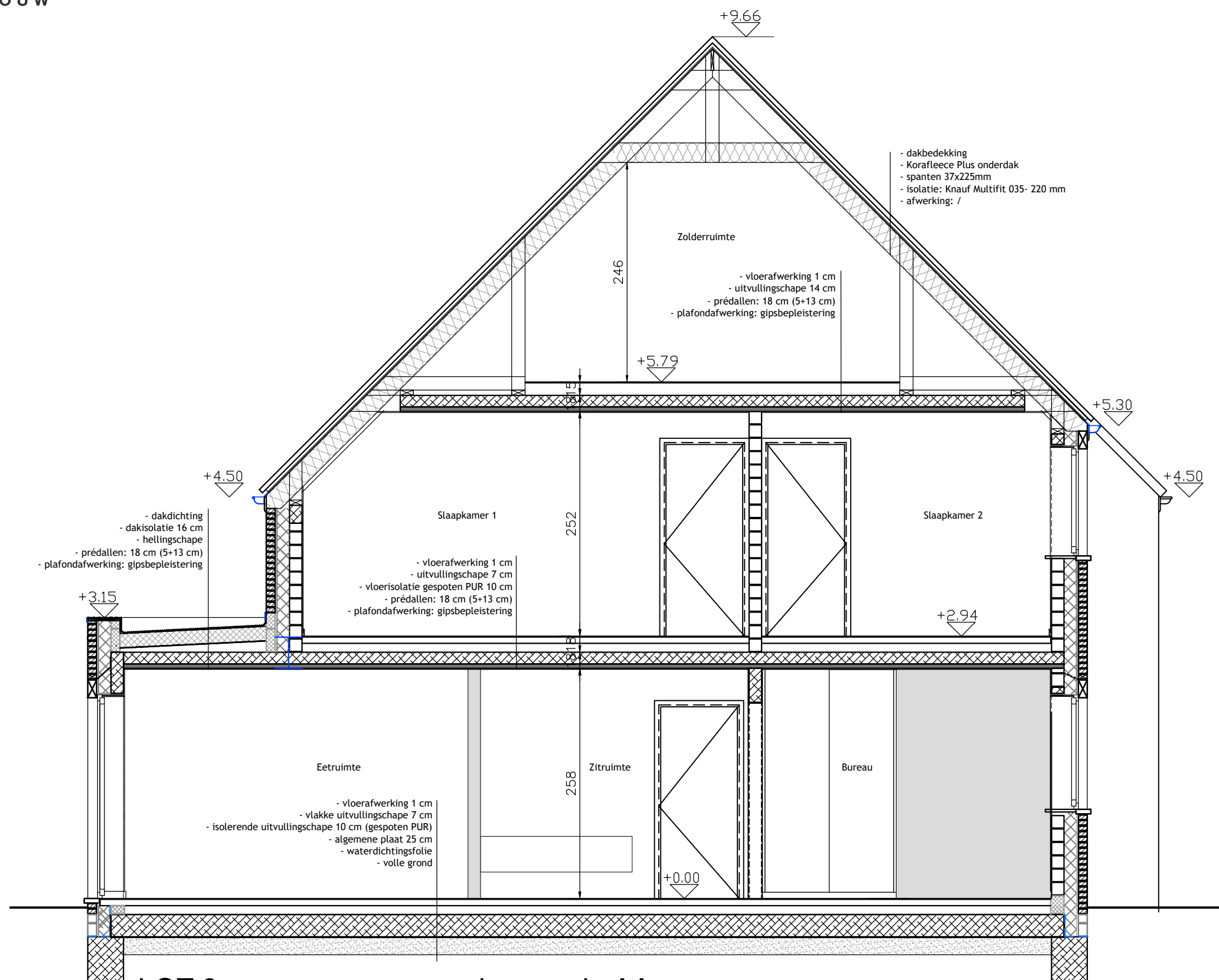
LOT 8 (Vogelzangstraat 2C) doorsnede AA schaal 1/50
