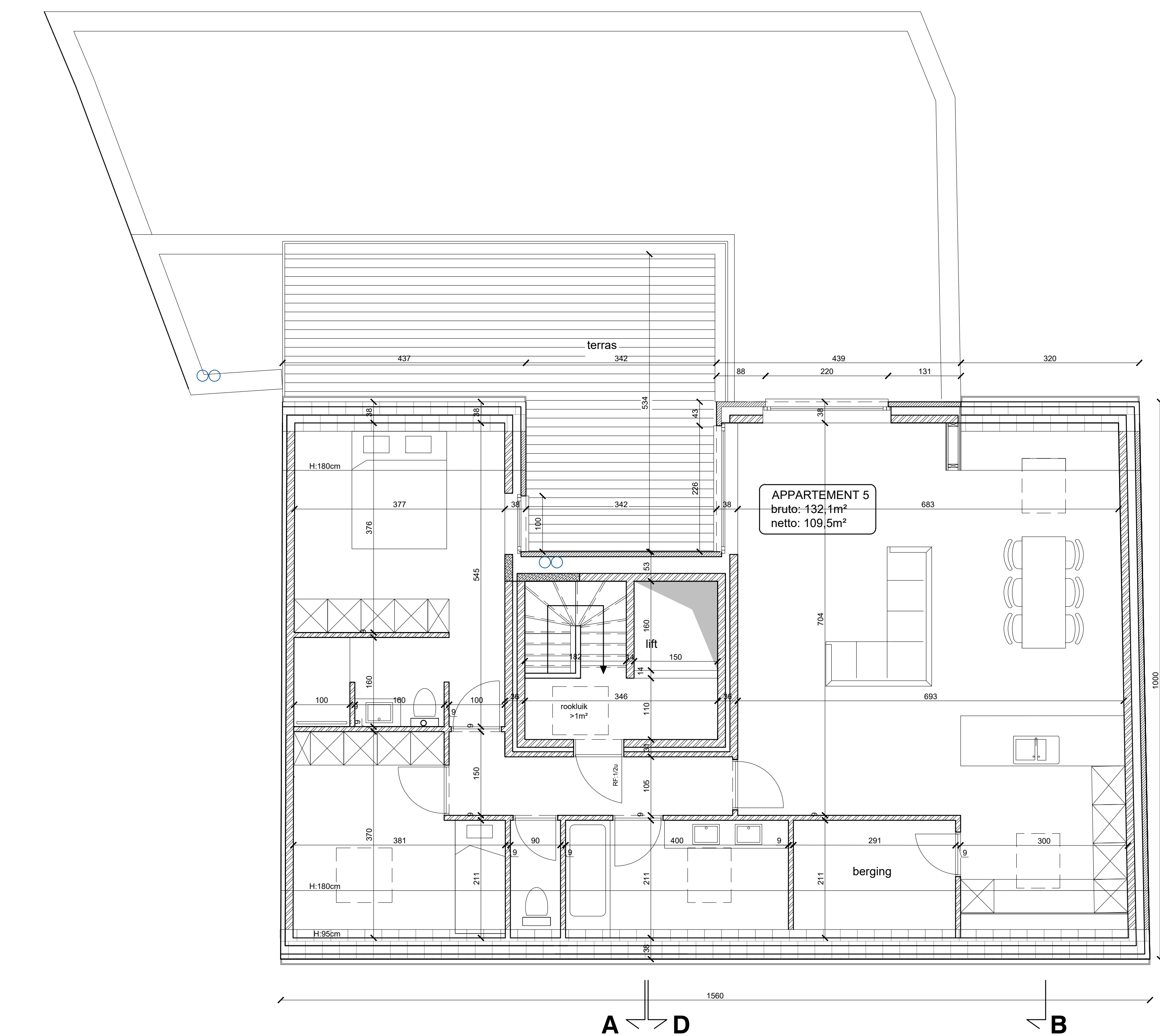
Tweede verdieping 1/50
