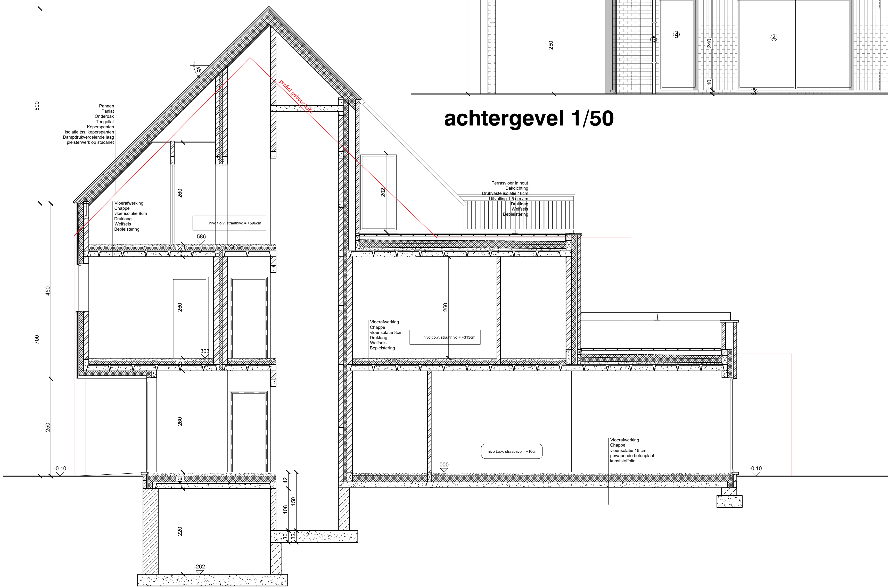
Doorsnede AA 1/50
