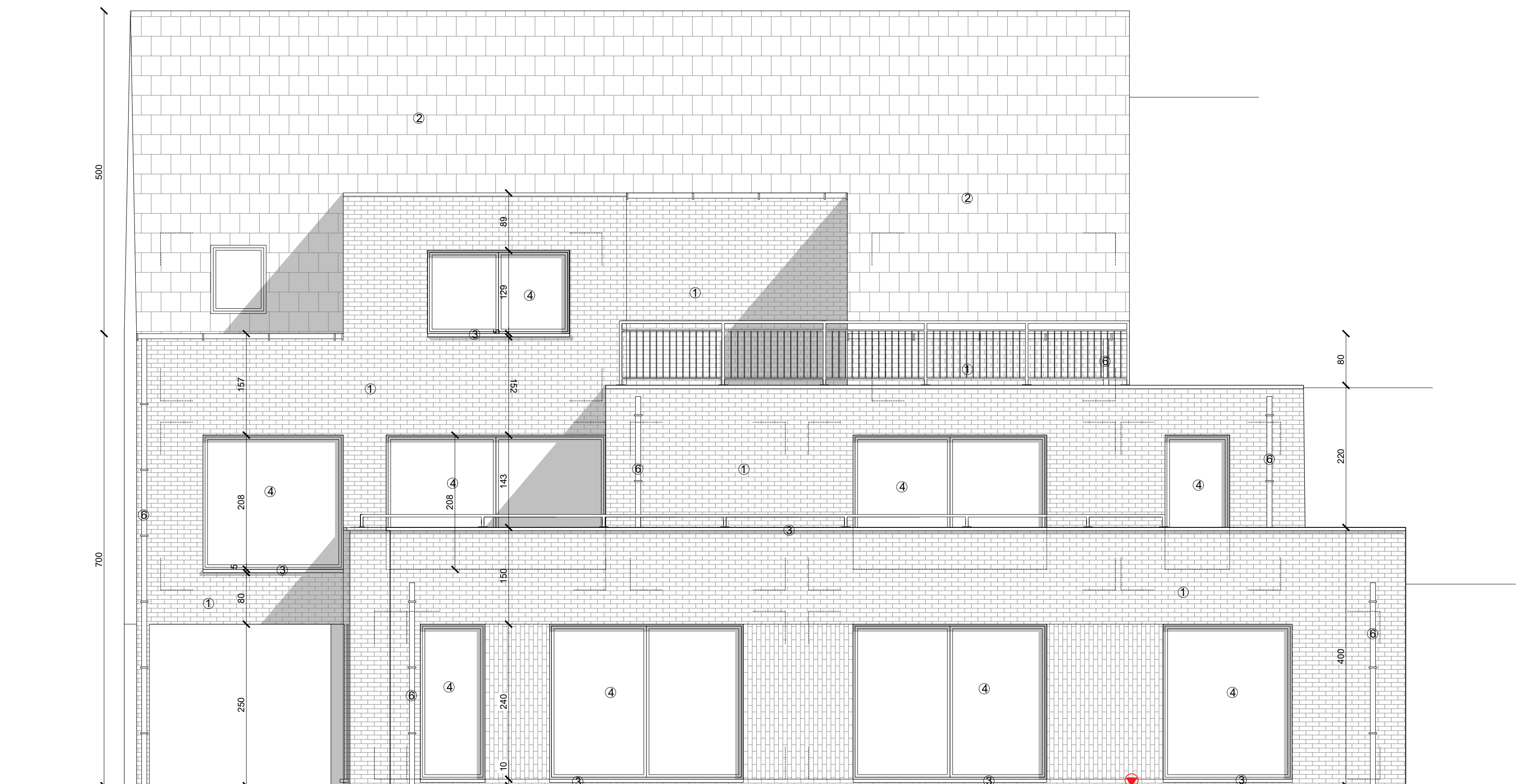
achtergevel 1/50
