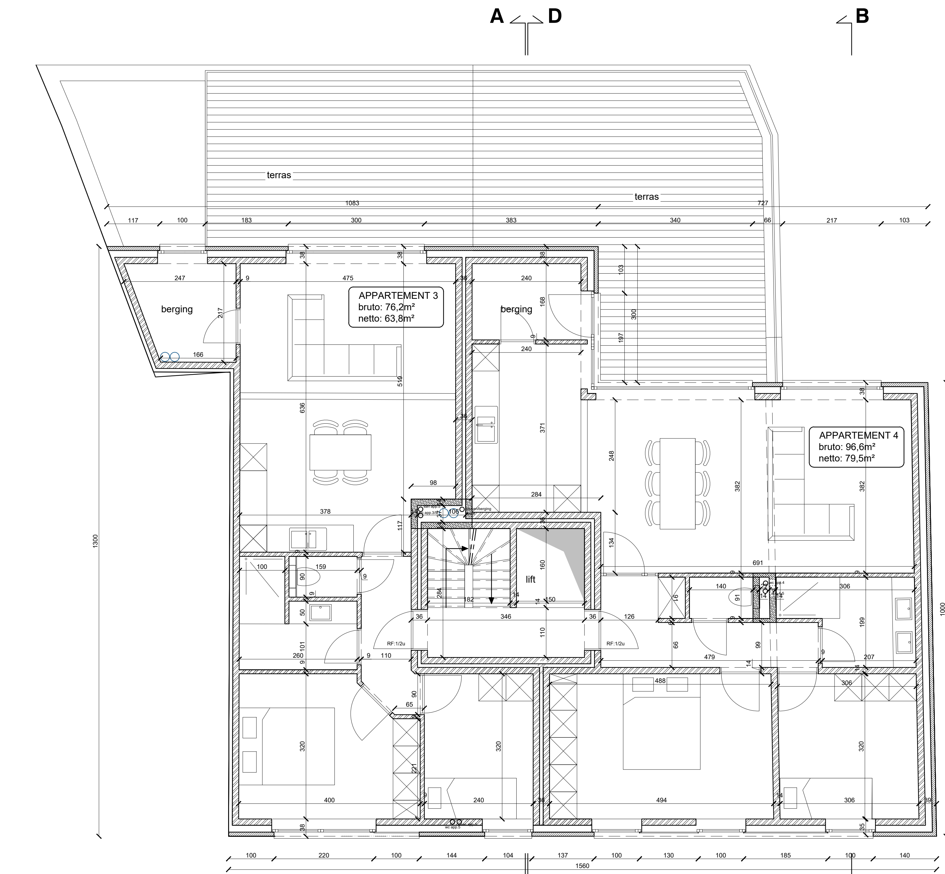
Eerste verdieping 1/50
