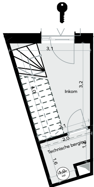
gelijkvloers
