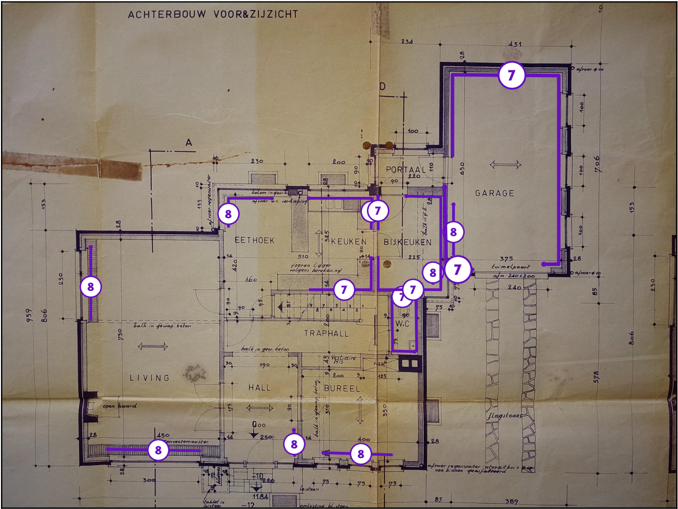
Legende van plan 1.6: Gelijkvloers plan 3
