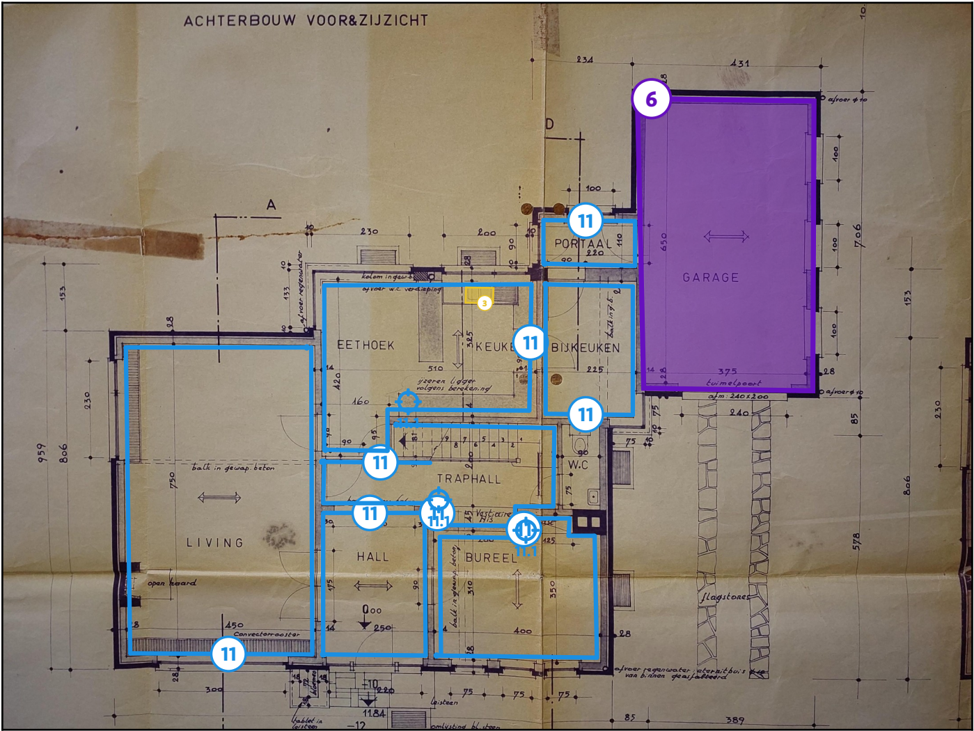
Legende van plan 1.3: Gelijkvloers plan
