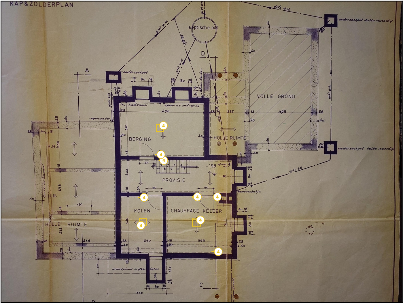
Legende van plan 1.2: Kelder plan 2
