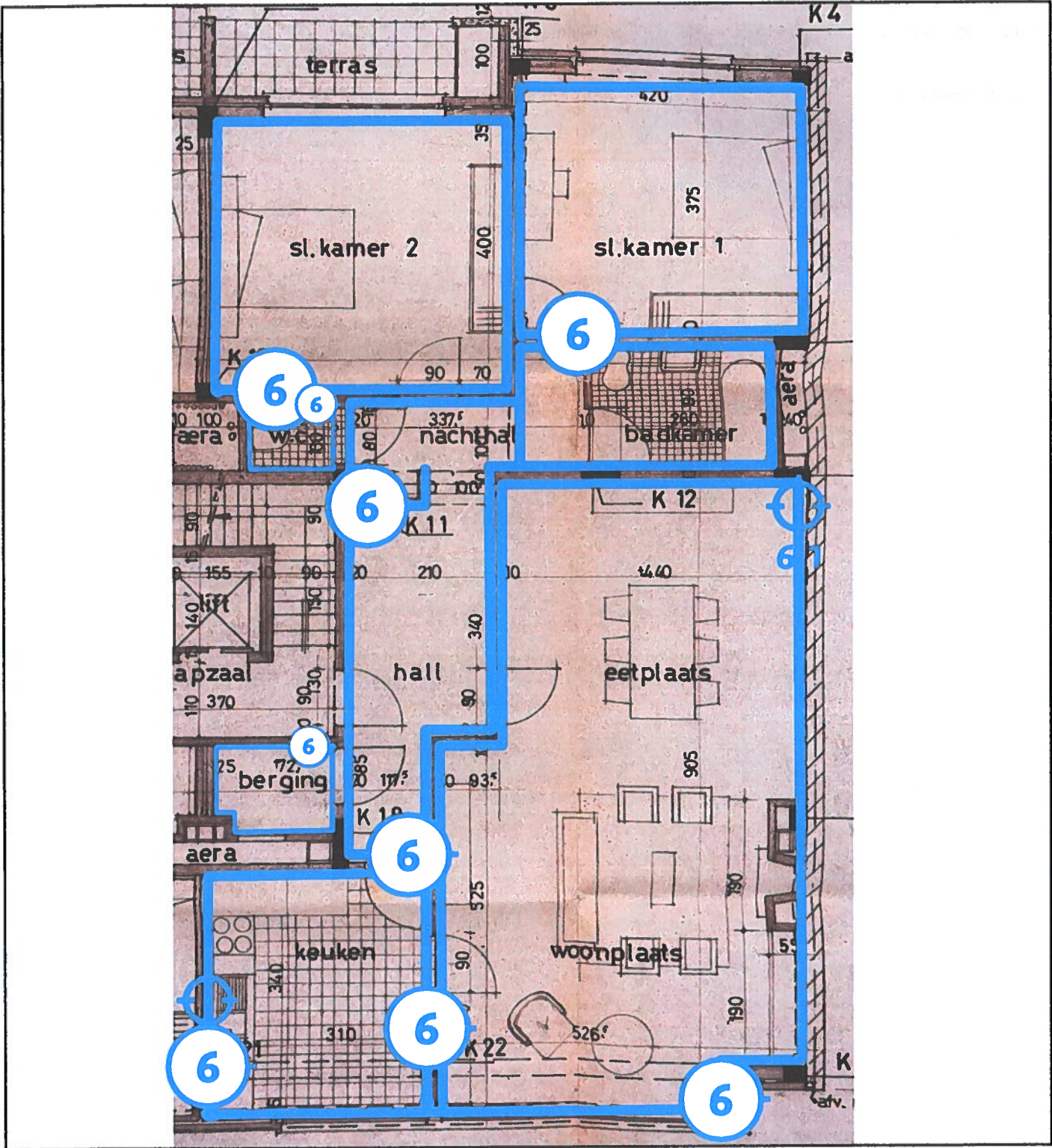
Legende van plan 1.5: Appartement niveau +2 - pleisterwerk wand
