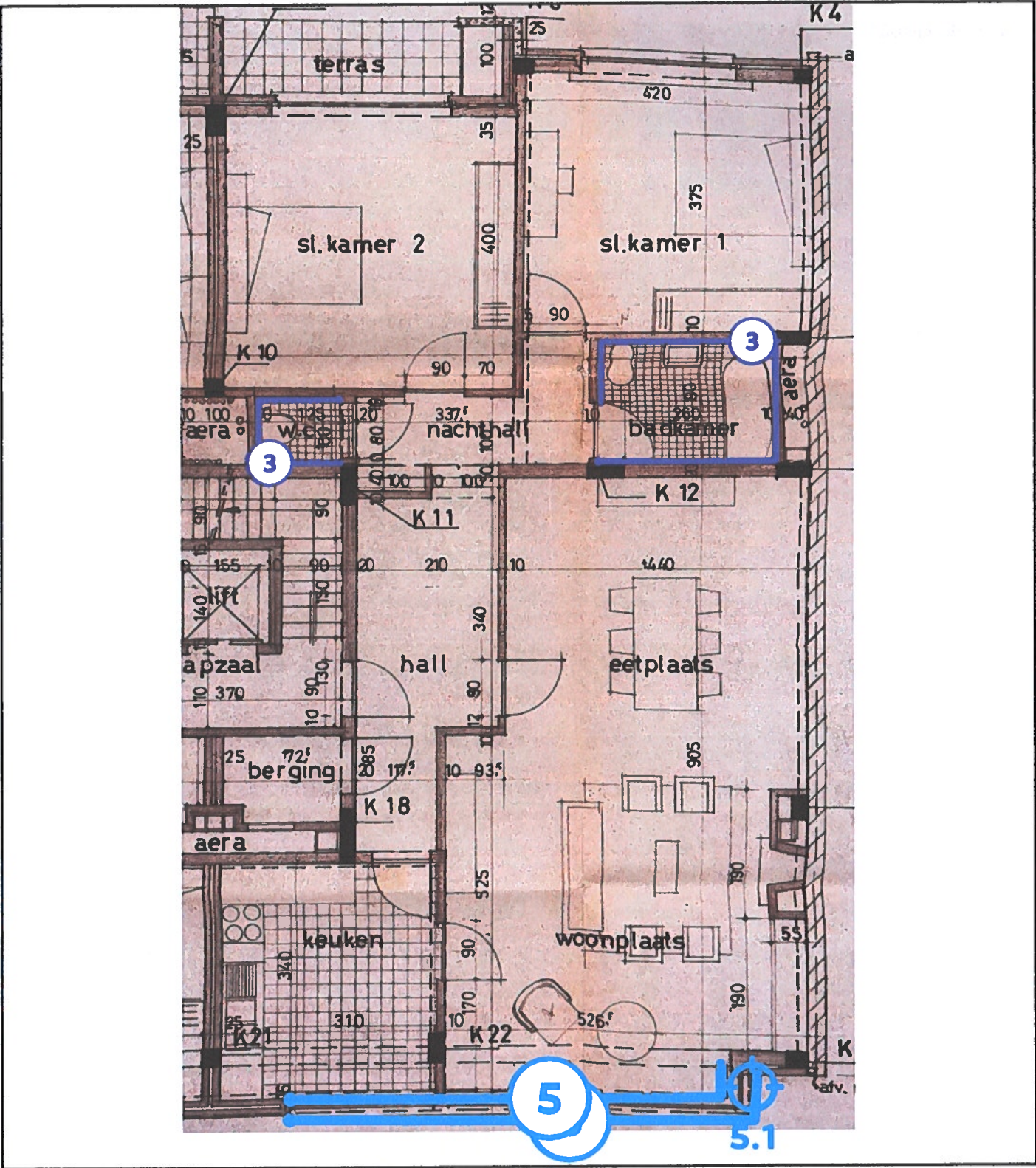
Legende van plan 1.4: Appartement niveau +2 - wandtegels - mastiek
