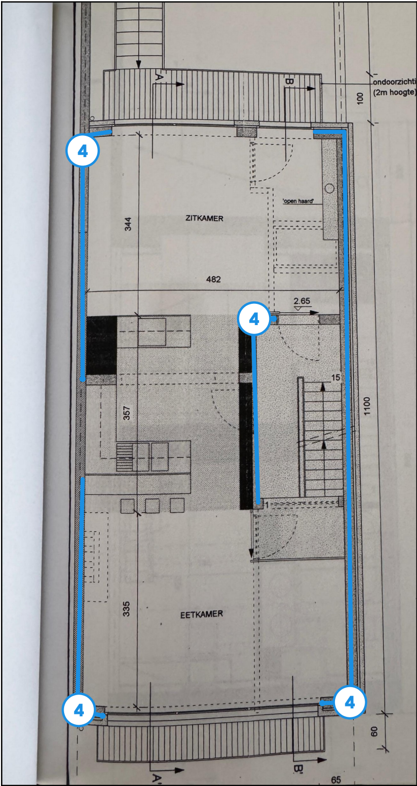
Legende van plan 1.3: 1ste verdiep
