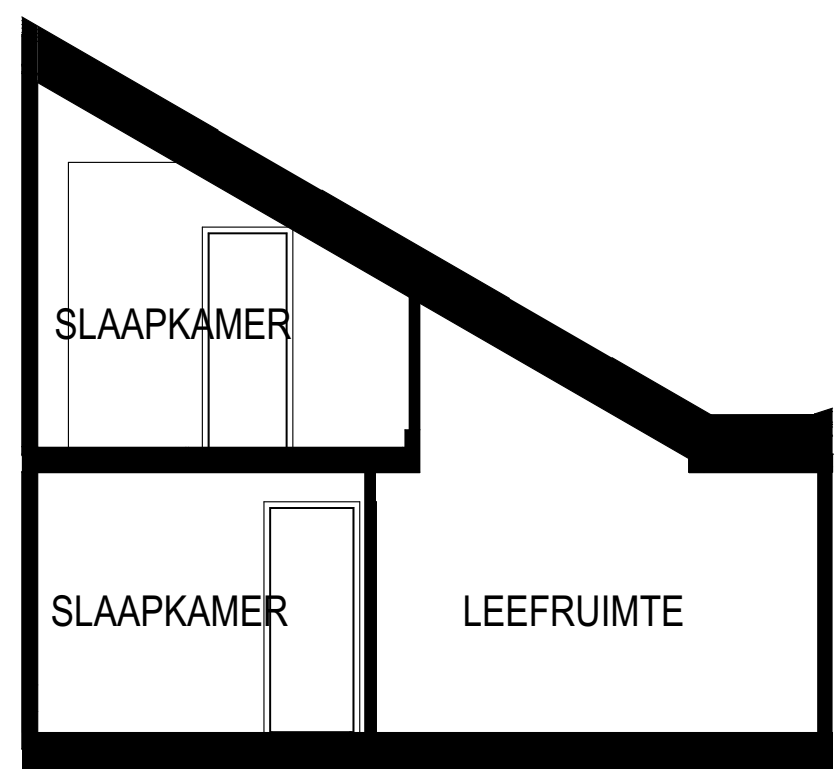
DOORSNEDE
