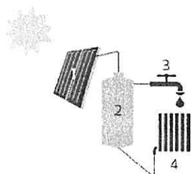
1. Zonnecollector | 2. Opslagvat voor warm water | 3. Sanitair warm water | 4. Verwarming Bij een zonnecollector op het dak wordt de zonnewarmte opgevangen en wordt deze via een leiding naar het opslagvat geleid. Het opslagvat is verbonden met het sanitair warm water en de verwarming.
