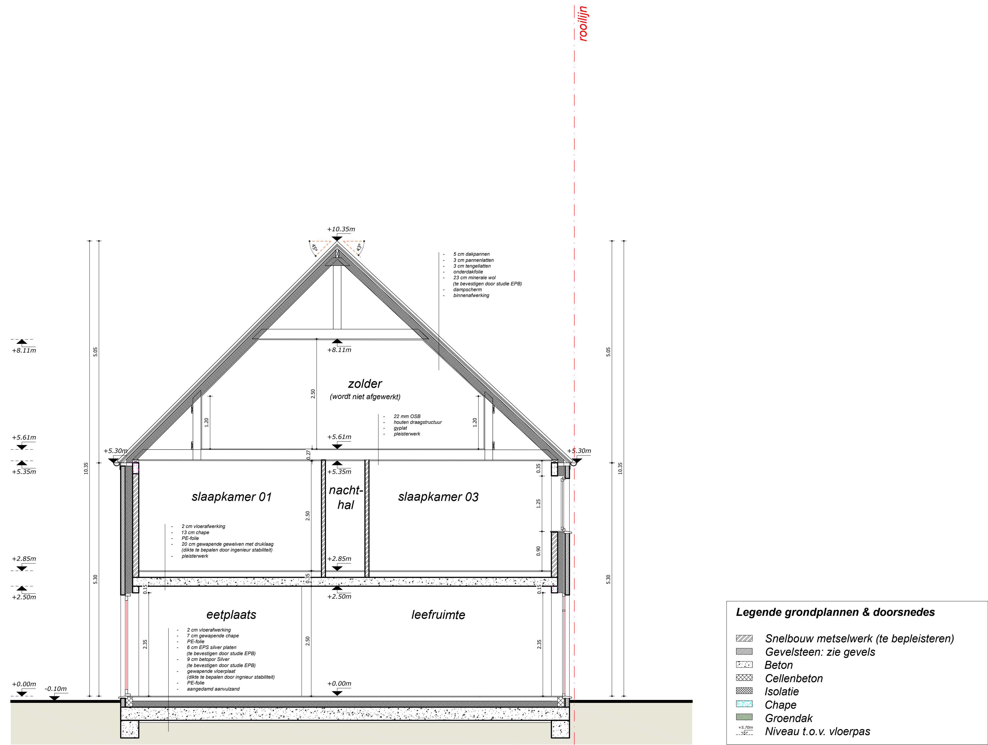
doorsnede BB' schaal 1:50
