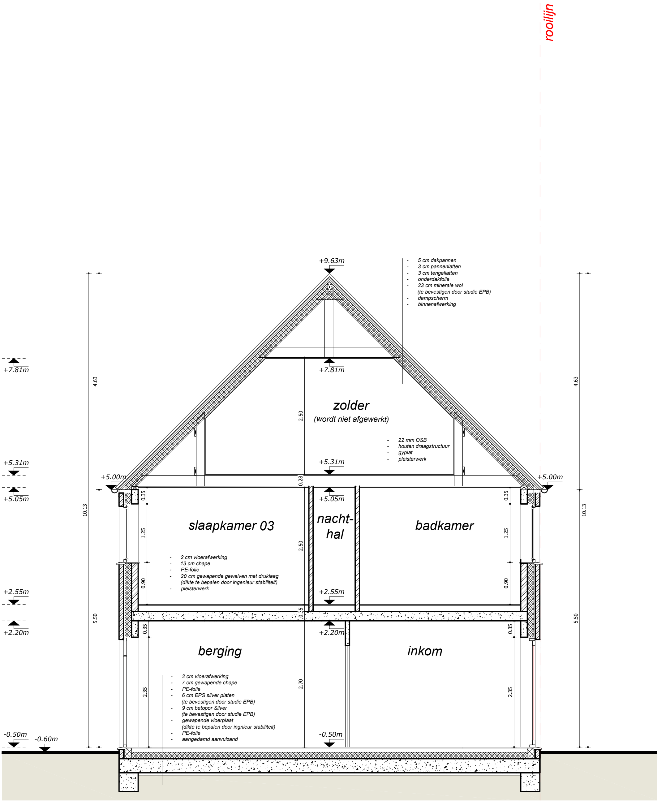
doorsnede GG' schaal 1:50
