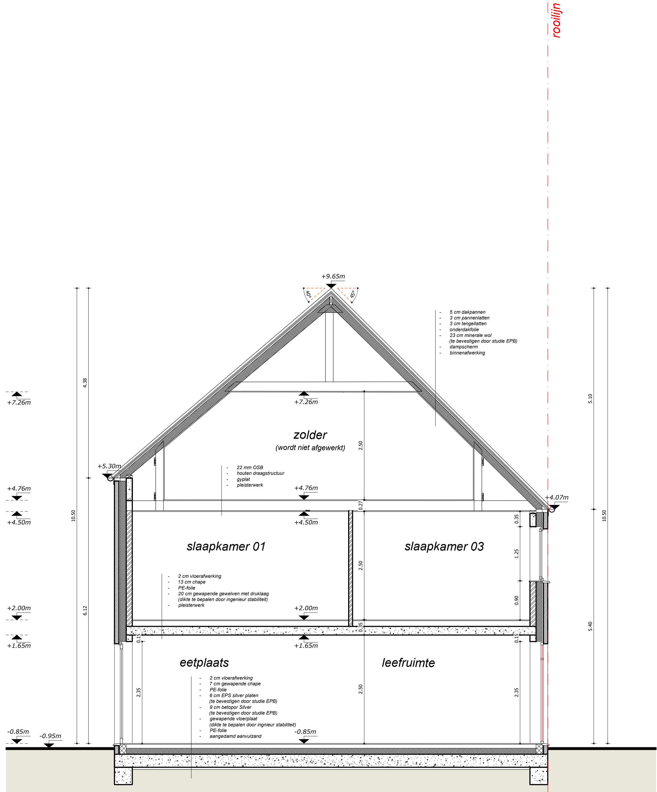
doorsnede JJ'
