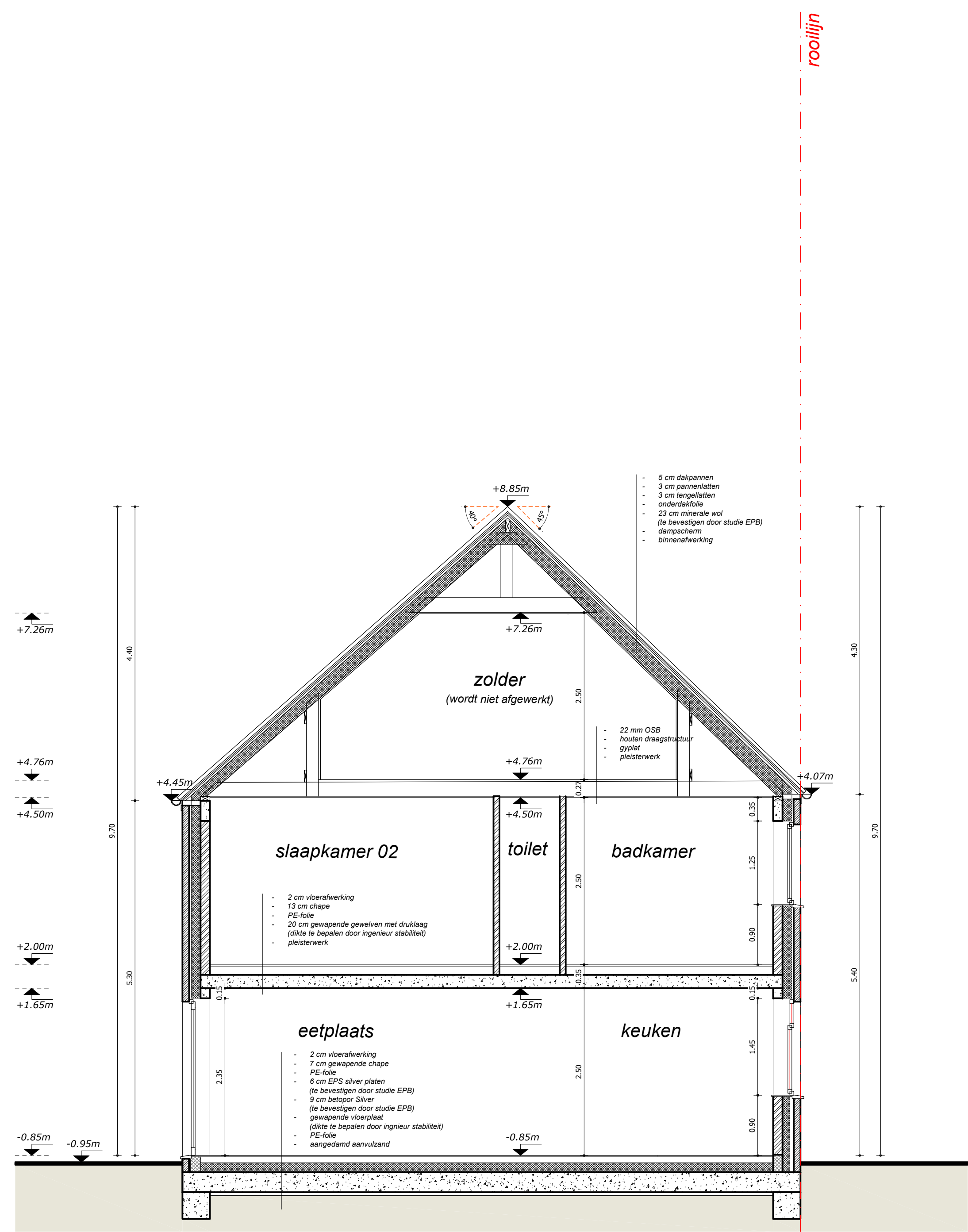
doorsnede KK' schaal 1:50
