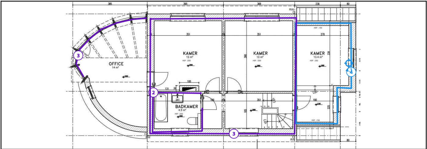
Legende van plan 1.5: Plan muren 1ste verdiep
