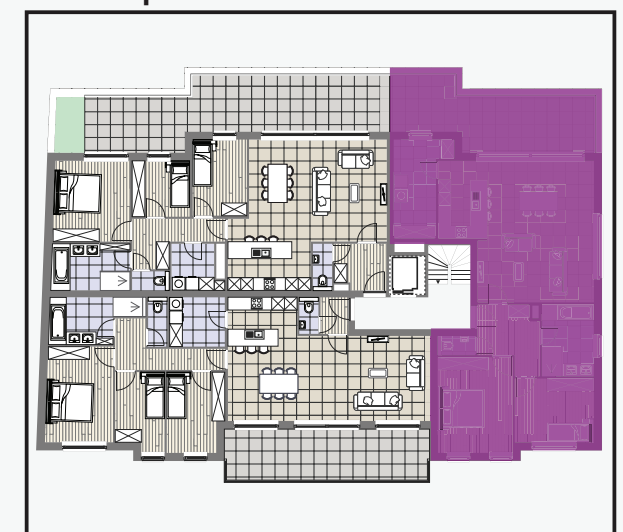
Grondplan
