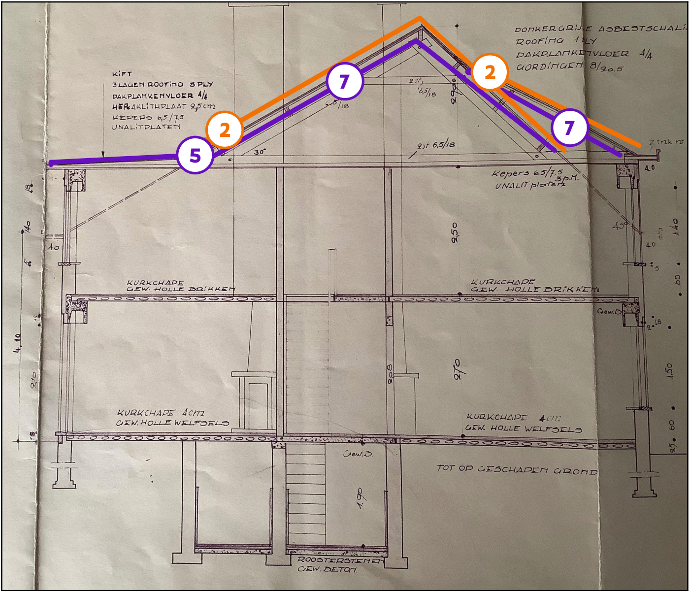
Legende van plan 1.5: Doorsnede
