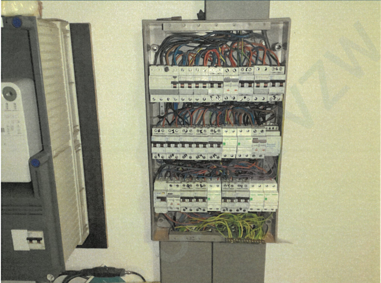
Elektrisch bord
