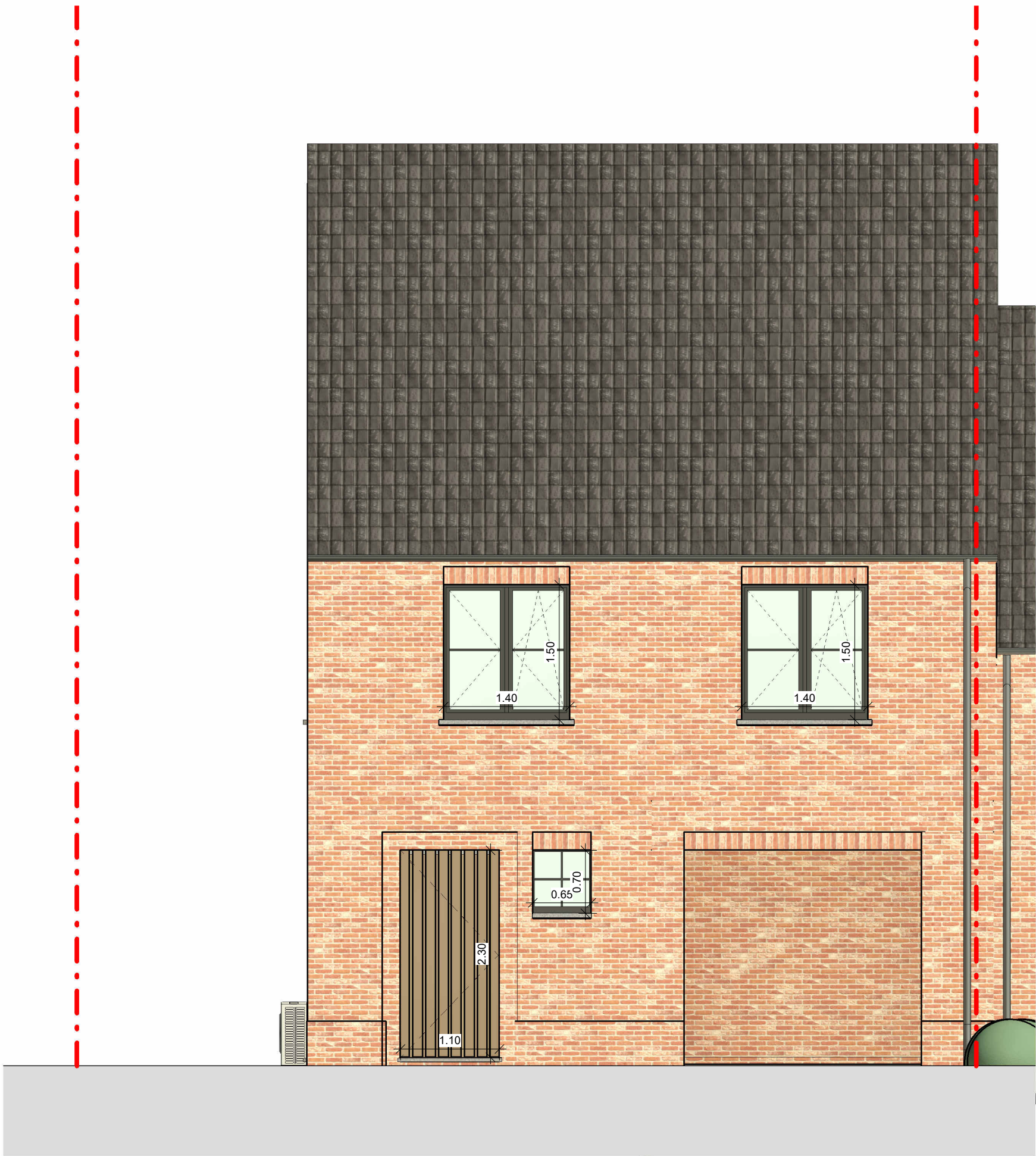
Voorgevel - Lot 4 1 : 50 0 1 2 3 4 5
