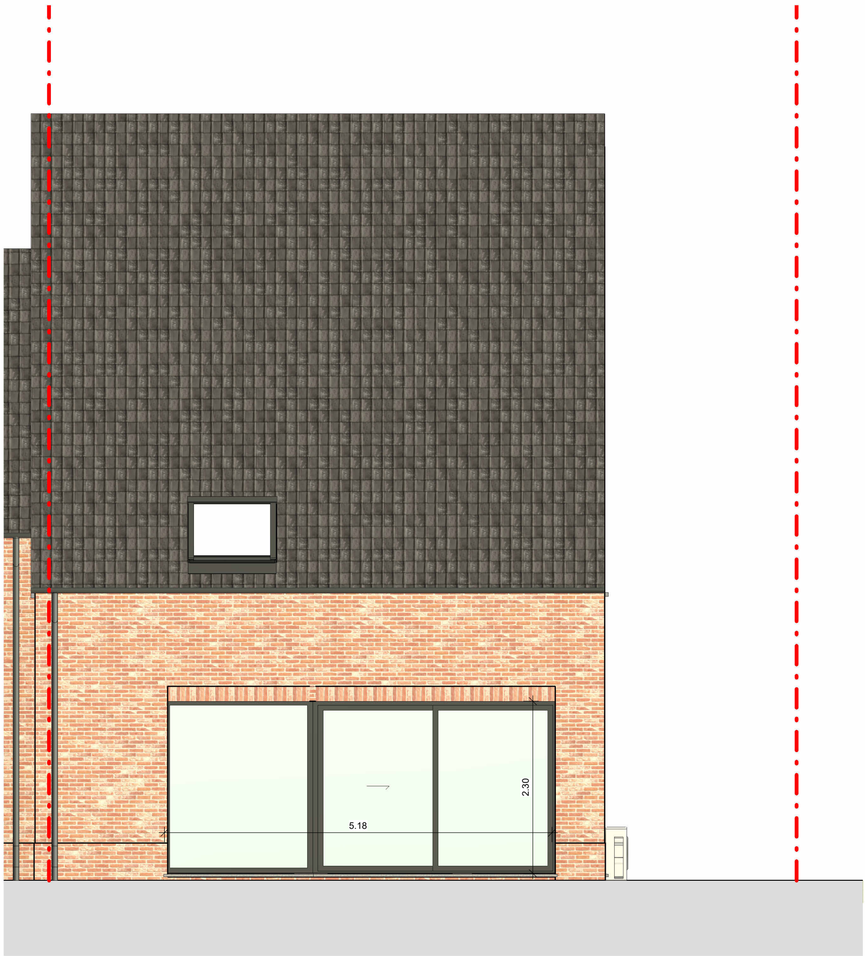
Achtergevel - Lot 4
