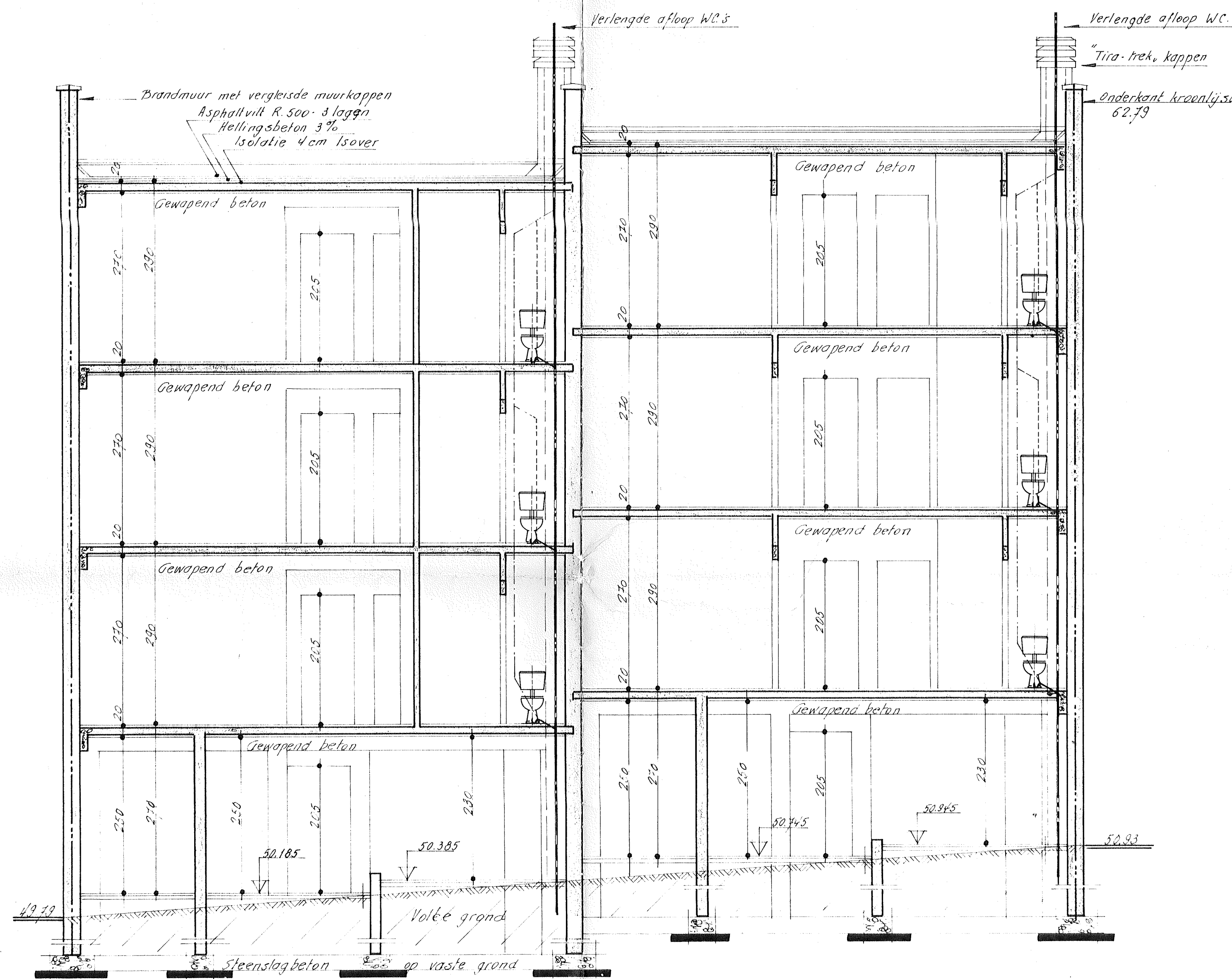
SNEDE B-B'
