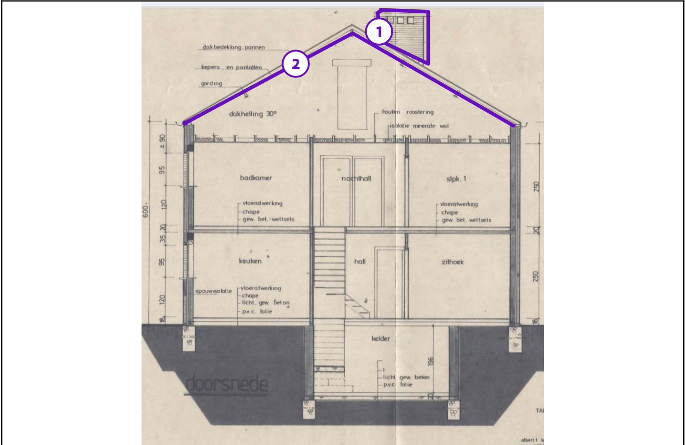
Legende van plan 1.6: Doorsnede
