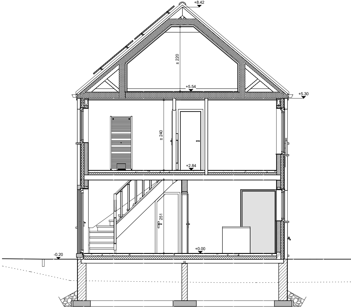
COUPE AA
