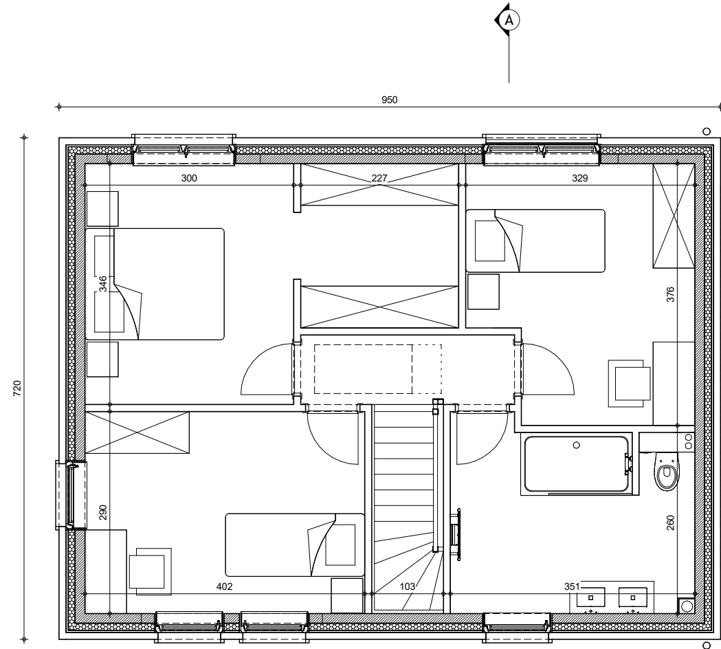
ETAGE
