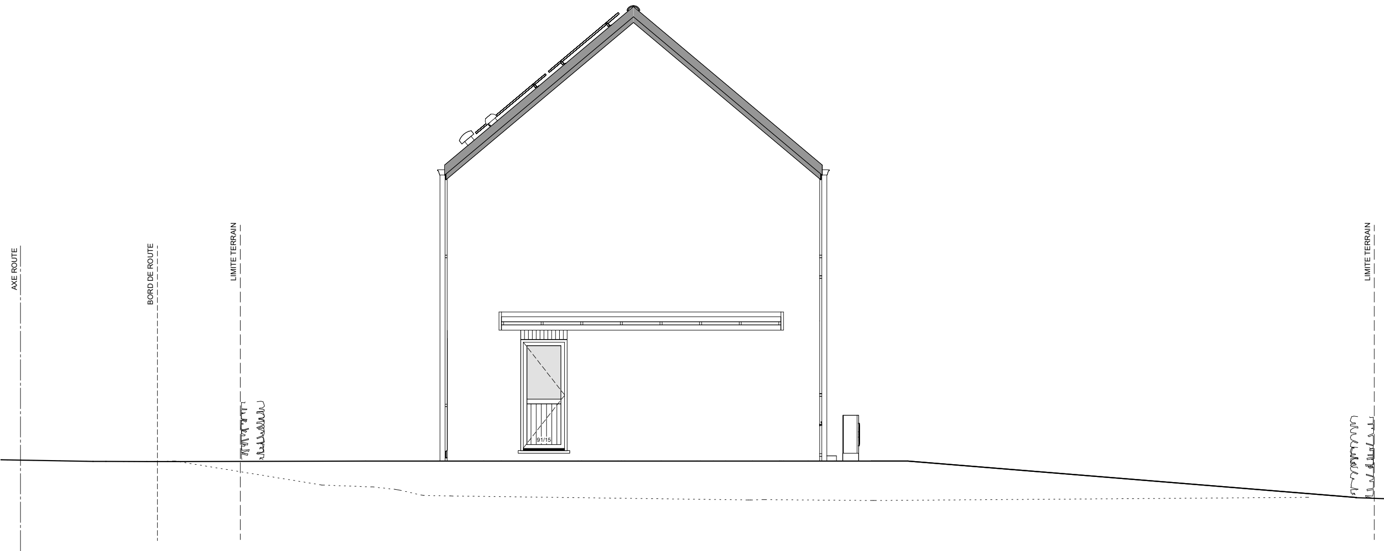
PIGNON DROIT
