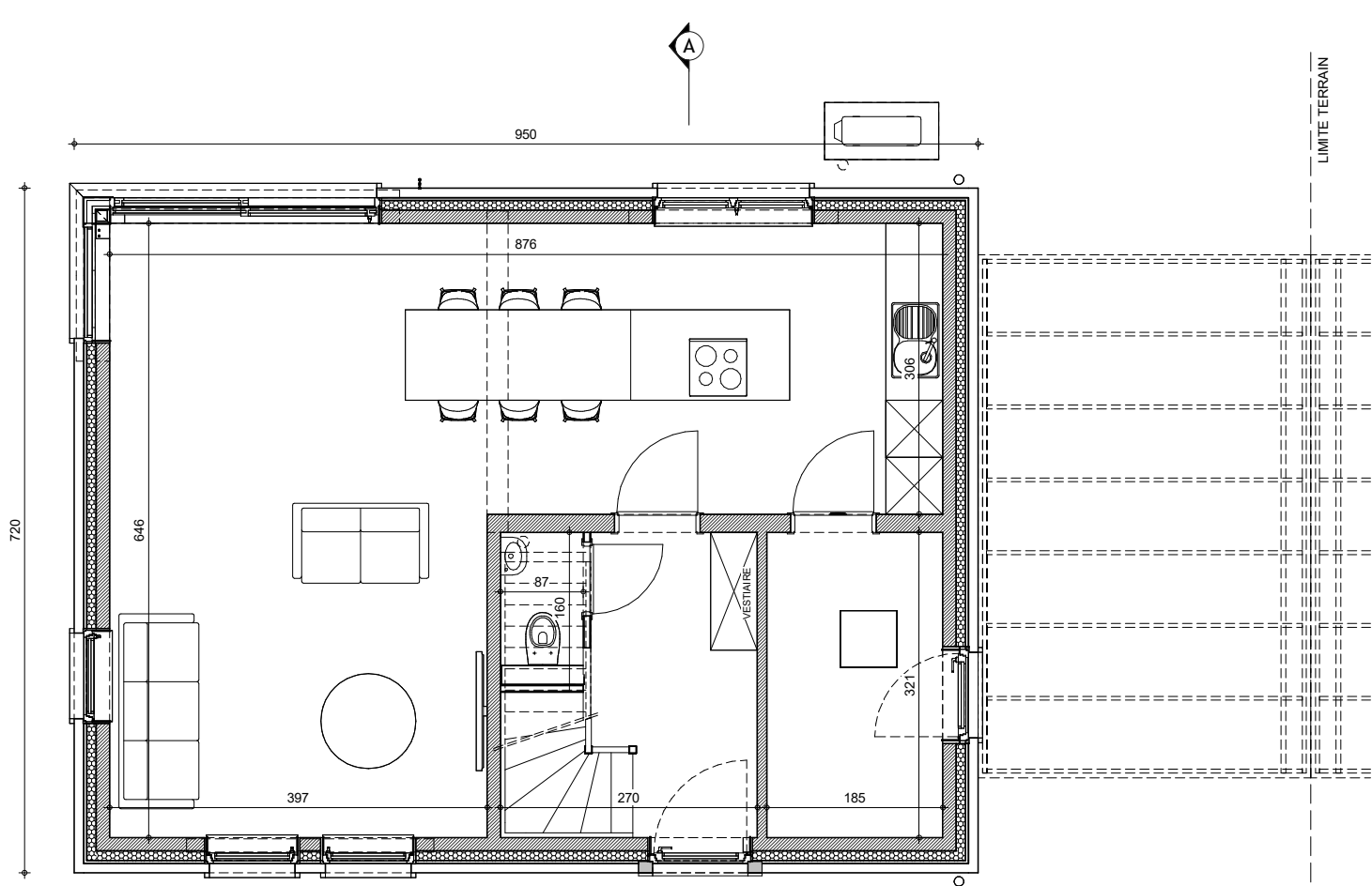
REZ-DE-CHAUSSEE
