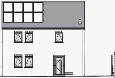
Façade avant
