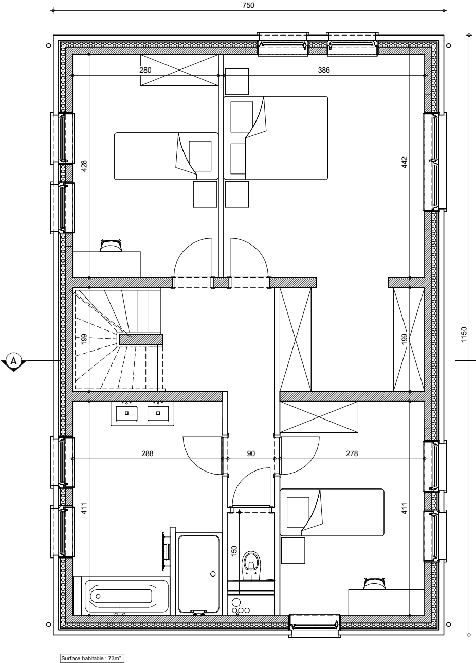
ETAGE 1
