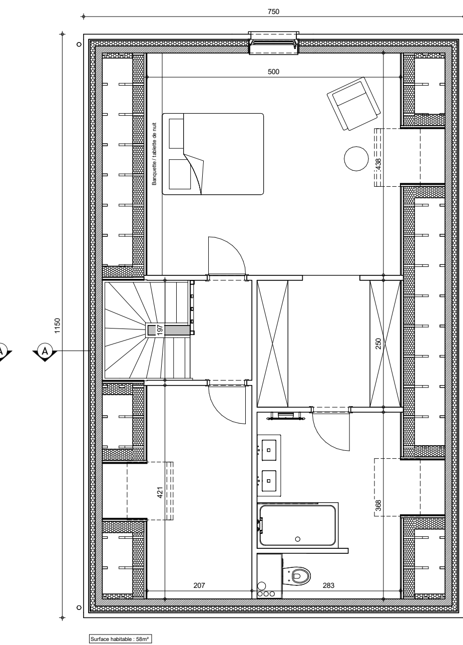
ETAGE 2
