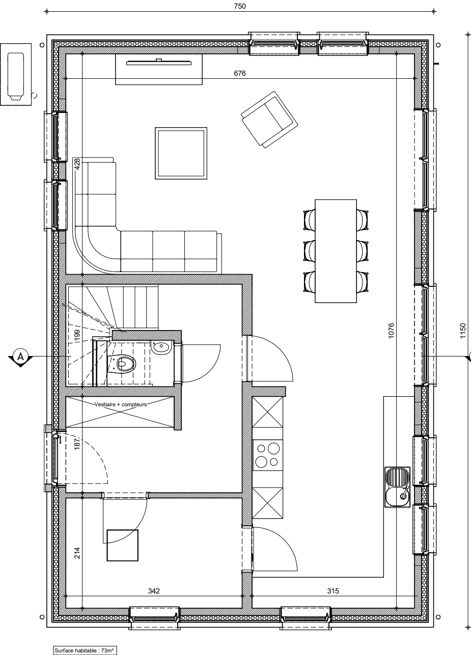
REZ-DE-CHAUSSEE
