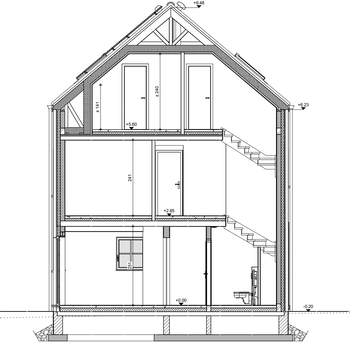
COUPE AA
