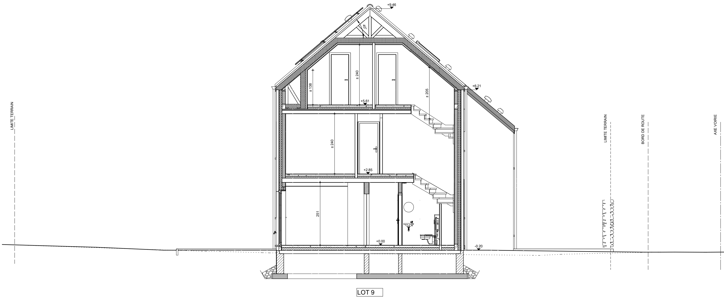
COUPE AA
