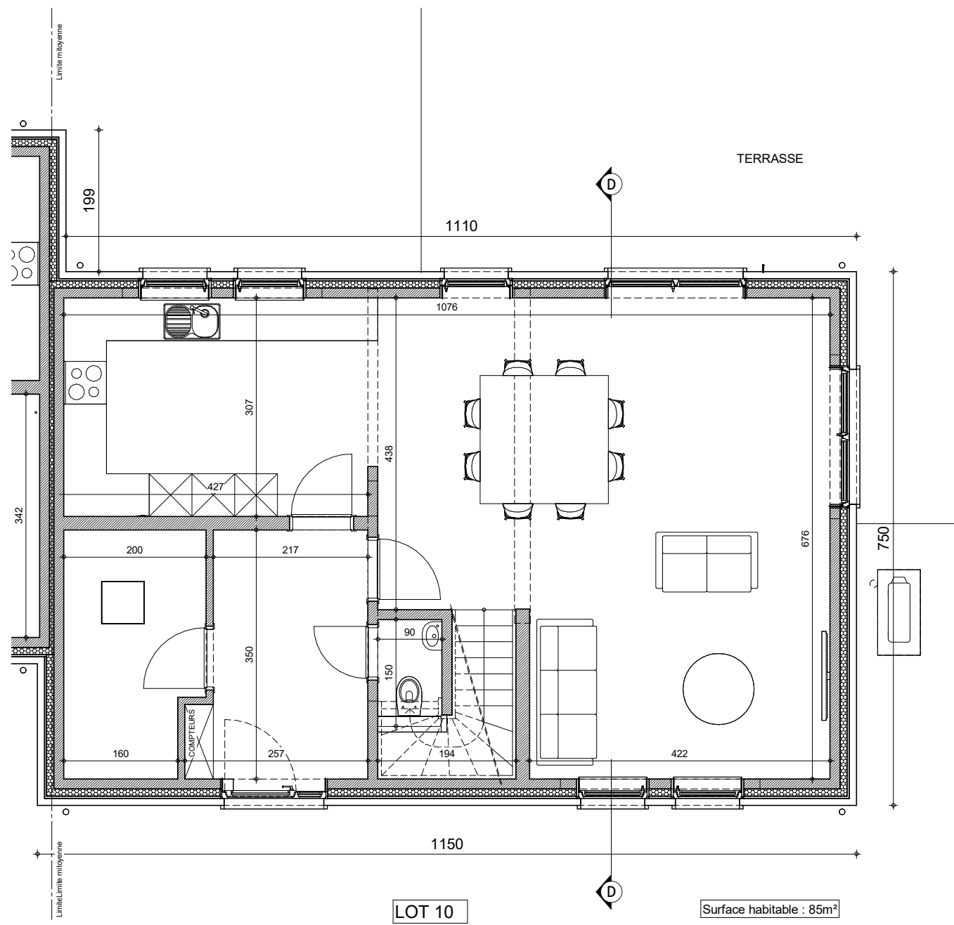
REZ-DE-CHAUSSEE
