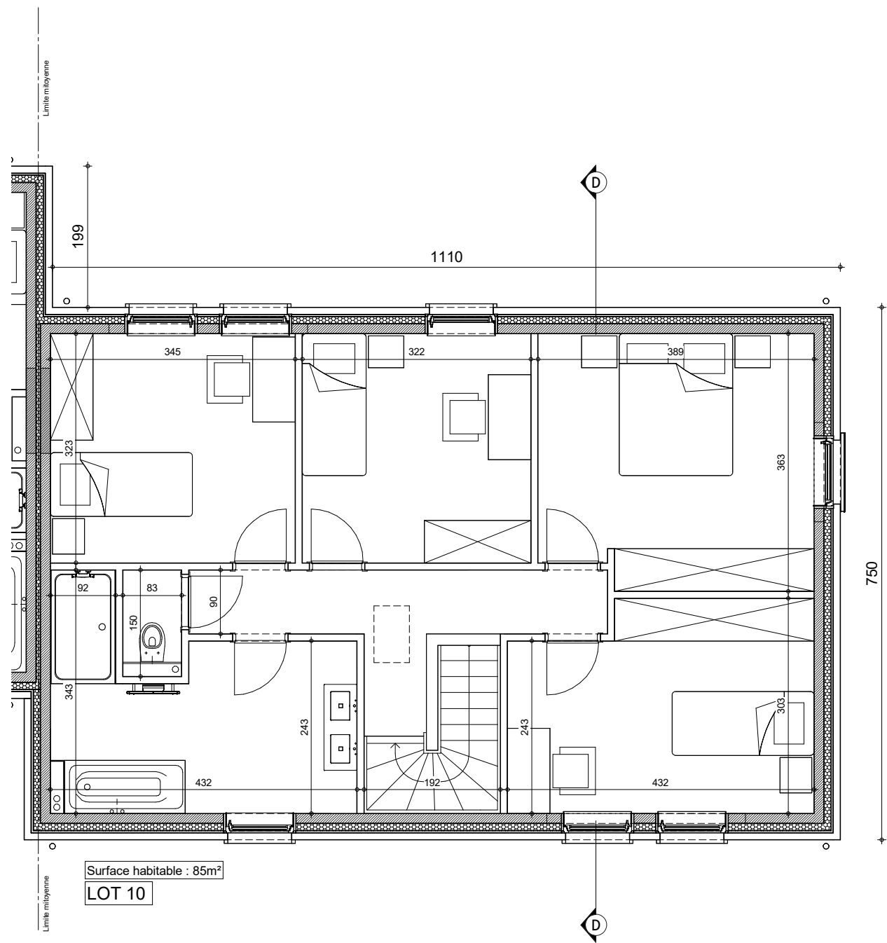
ETAGE
