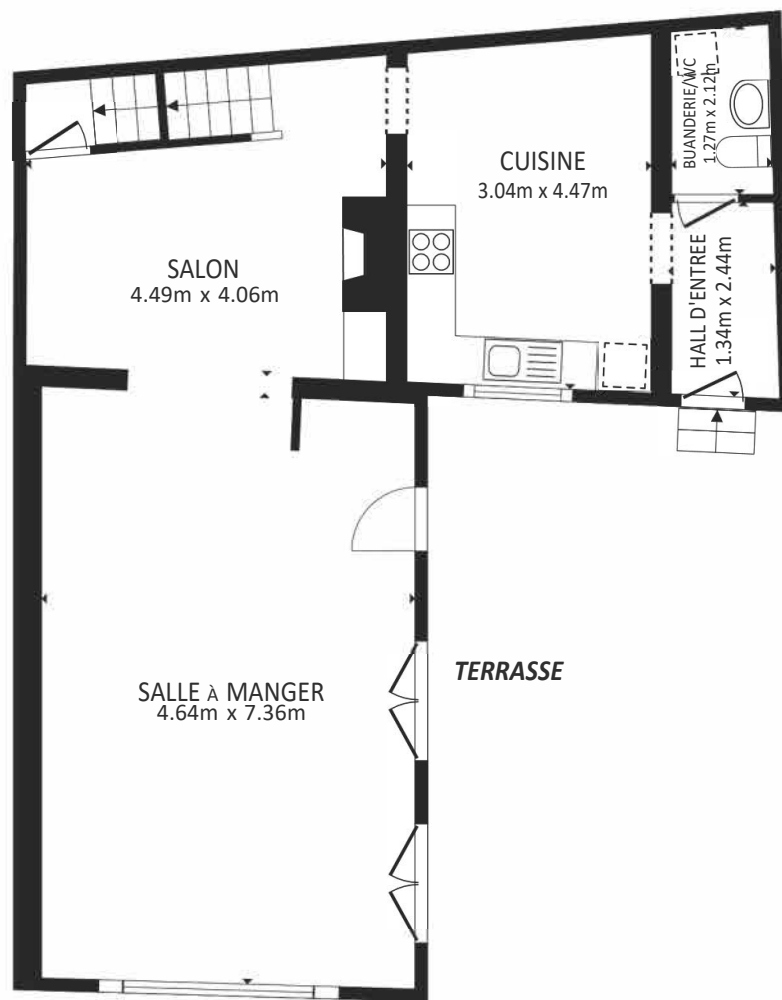
REZ-DE-CHAUSSEE
