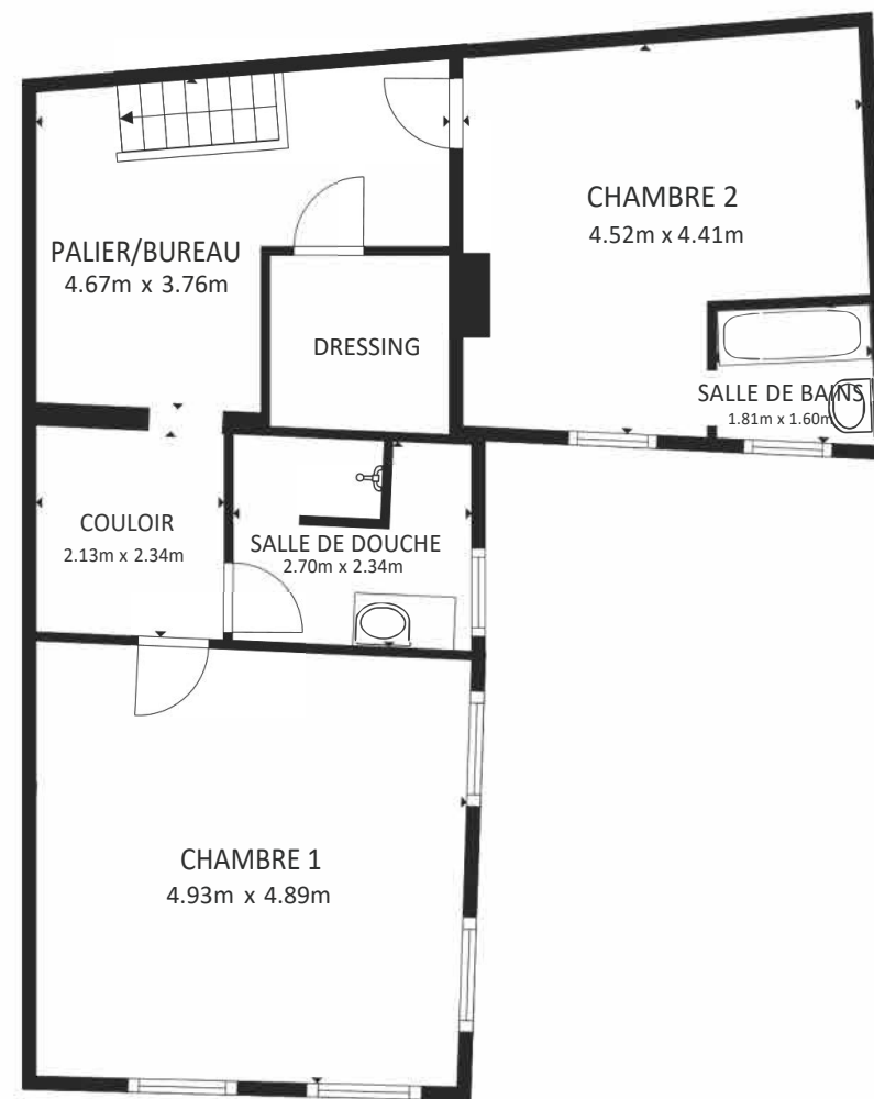
1ER ETAGE
