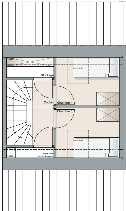
Grenier: variante 2 (non comprise)
