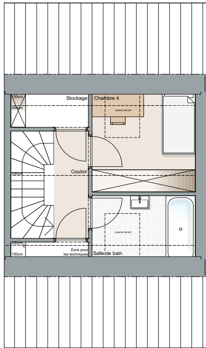
Grenier: variante 1 (non comprise)
