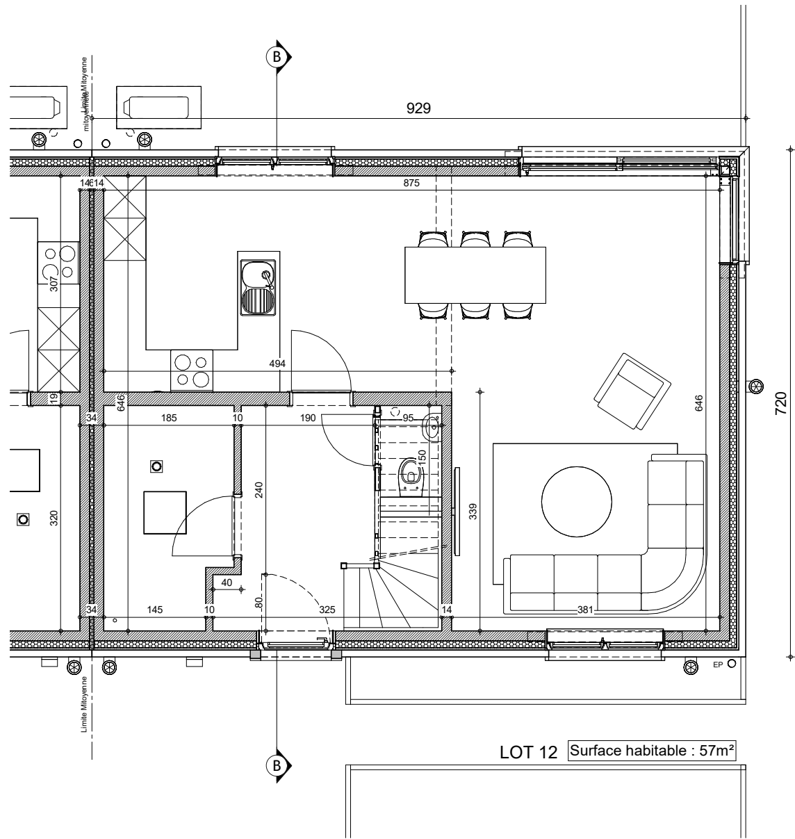
REZ-DE-CHAUSSEE
