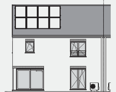
Façade arrière
