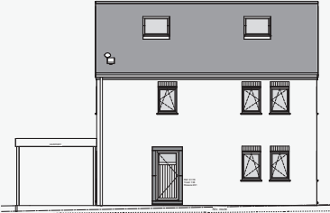
Façade avant
