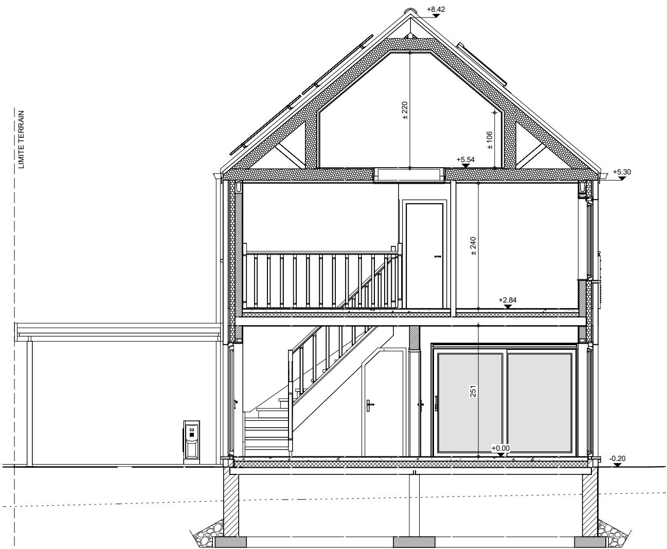
COUPE AA
