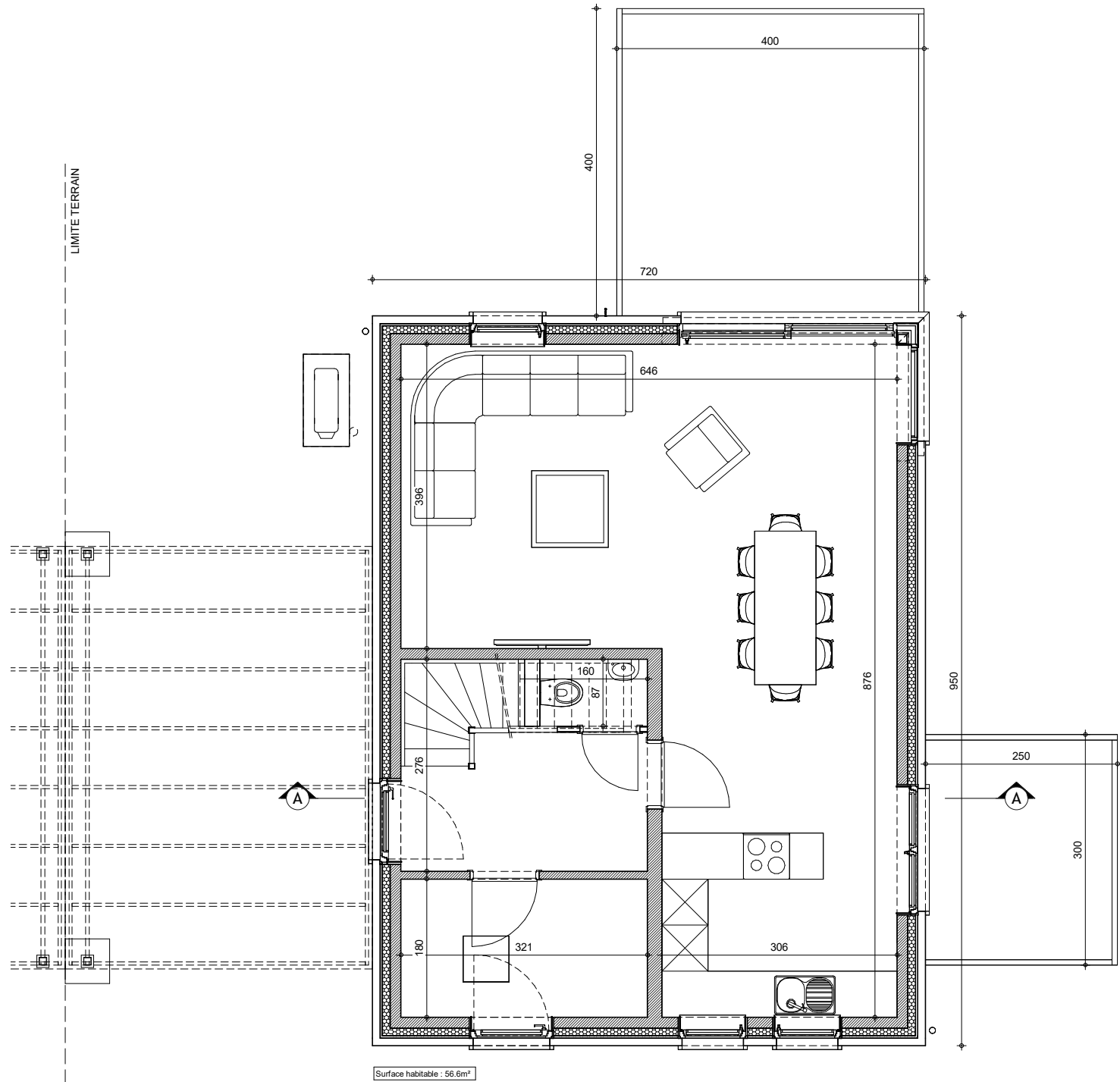
REZ-DE-CHAUSSEE
