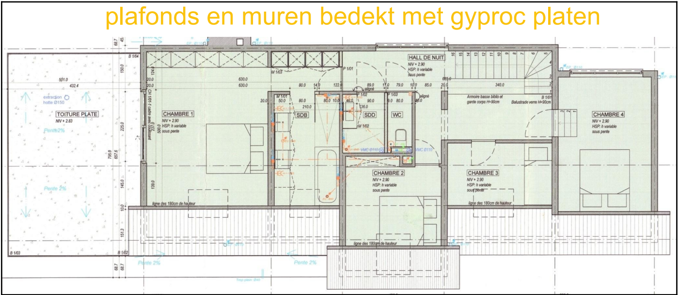
Legende van plan 1.5: Eerste verdieping (pleisterwerk)
