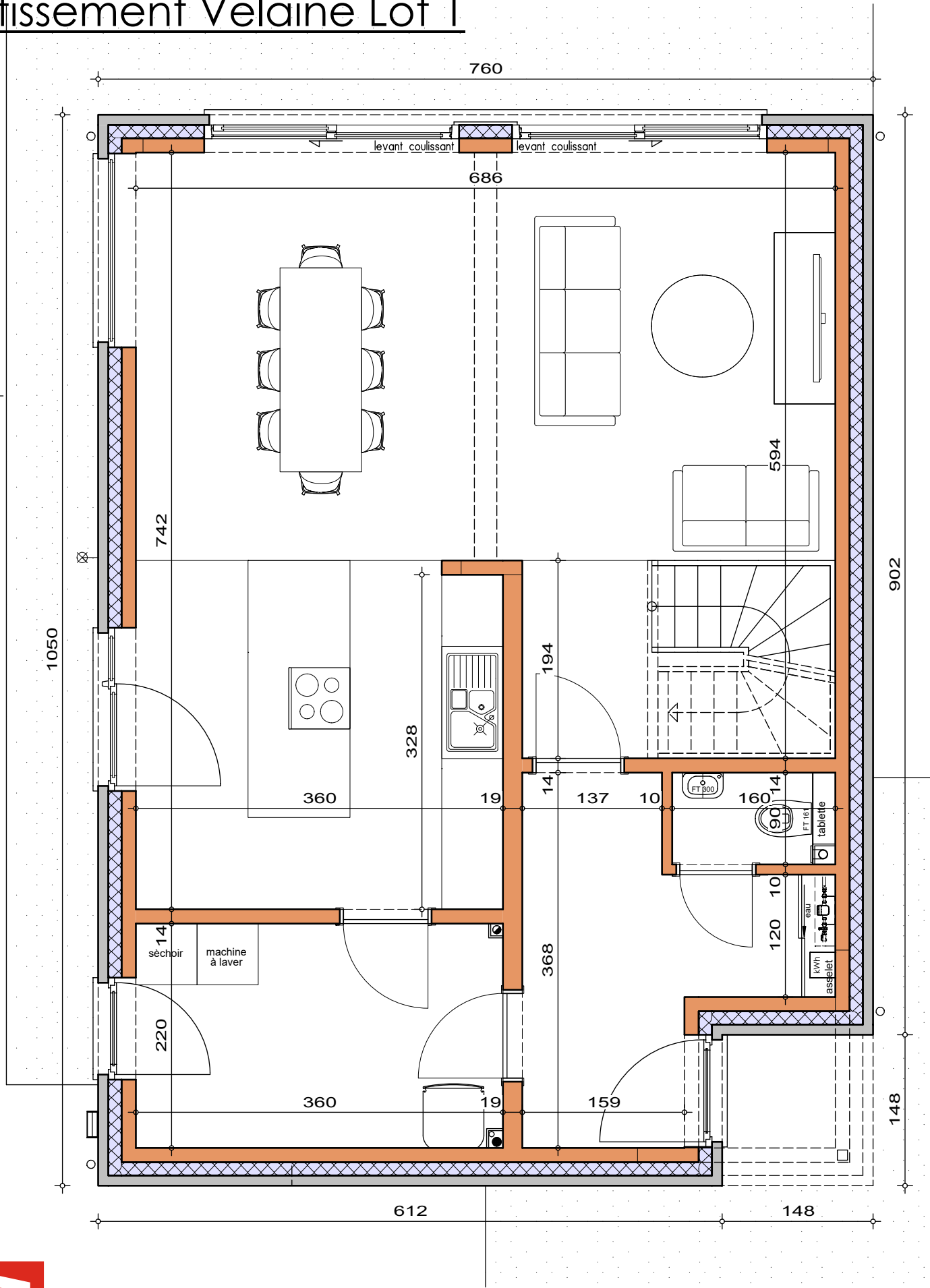
Rez de Chaussée Surface :77.61m 2
