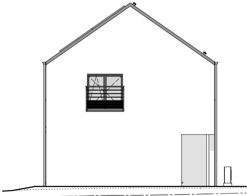
Pignon Avant
