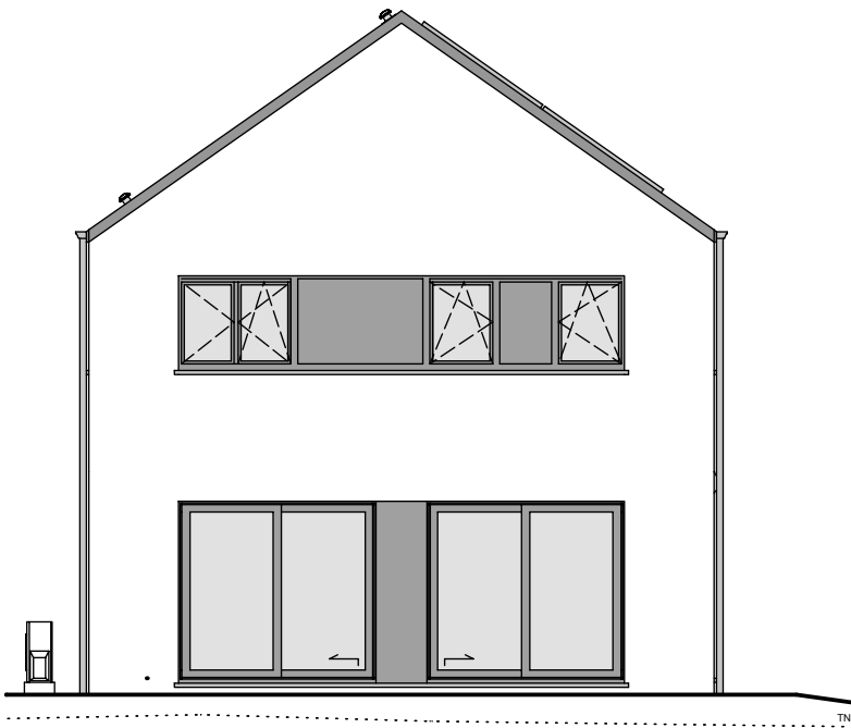
Pignon Arrière
