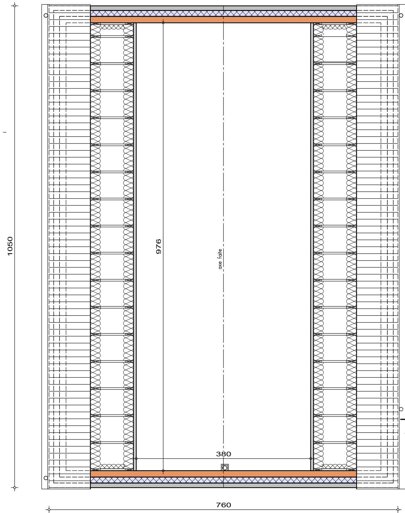
2ème ETAGE Surface :37.09m²
