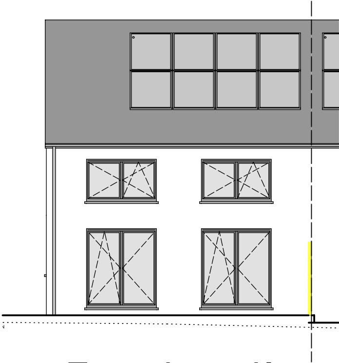
Façade arrière
