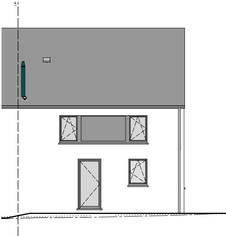
Façade avant
