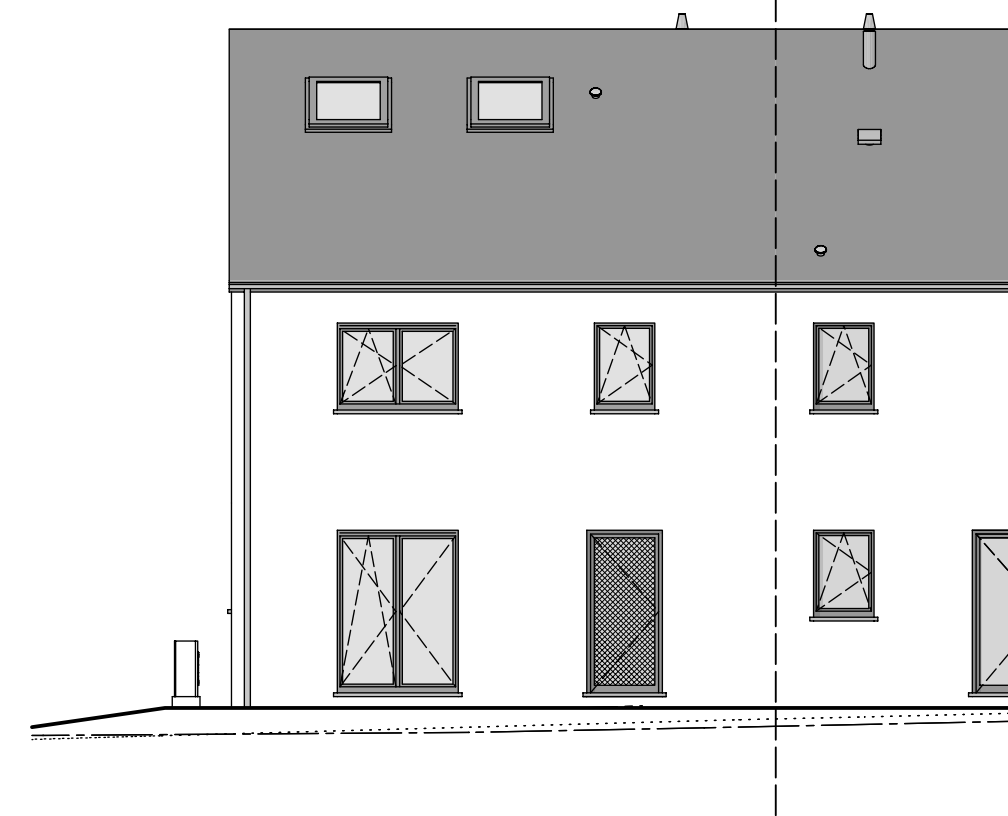
Façade avant
