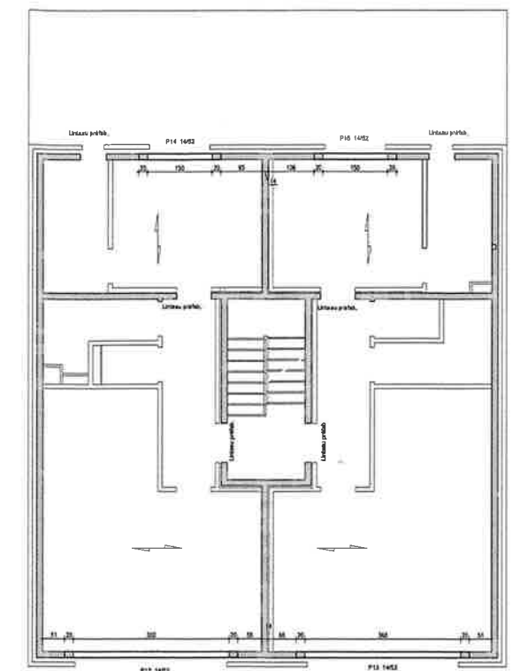
HAUT ETAGE
