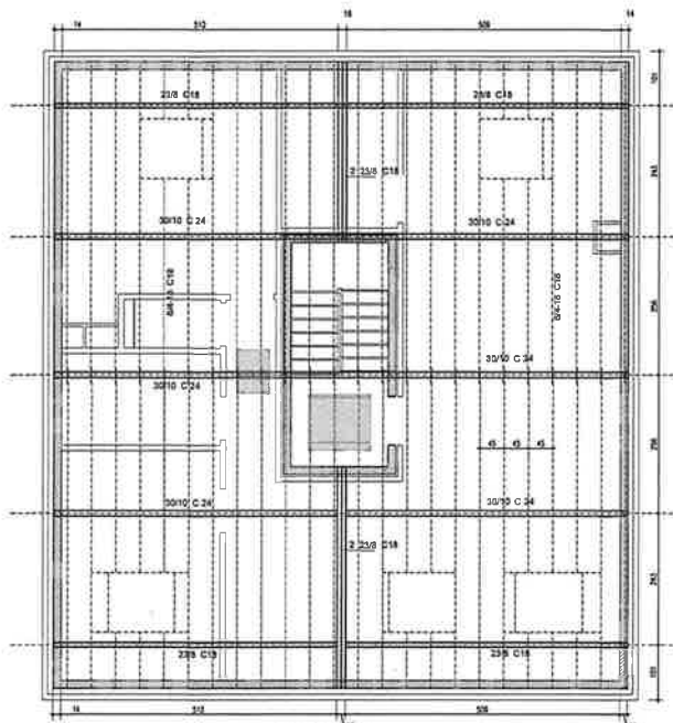
TOITURE
