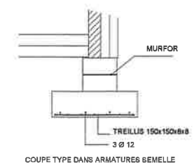
COUPE TYPE DANS ARMATURES SEMELLE
