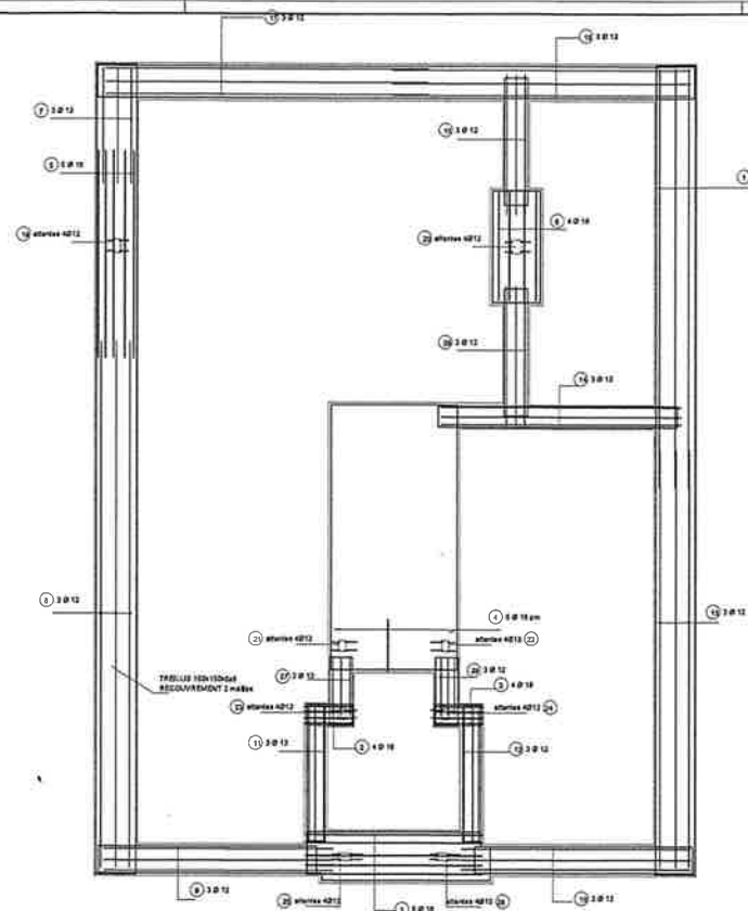
FONDATIONS armatures
