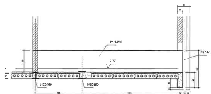
COUPE B-B
