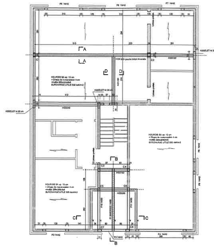
HAUT REZ-DE-CHAUSSEE
