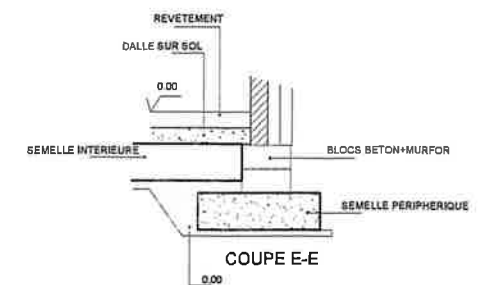
COUPE TYPE DANS ARMATURES SEMELLE
