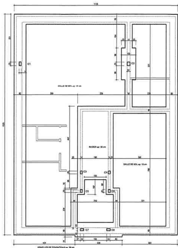
FONDATIONS
