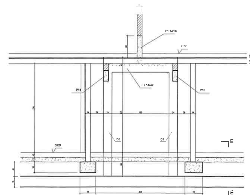
COUPE C-C
