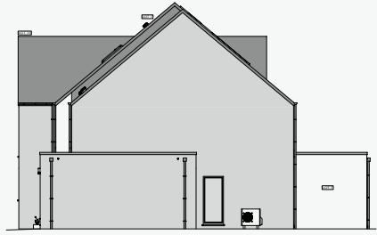
Pignon droit
