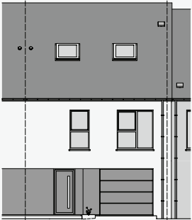
Façade avant
