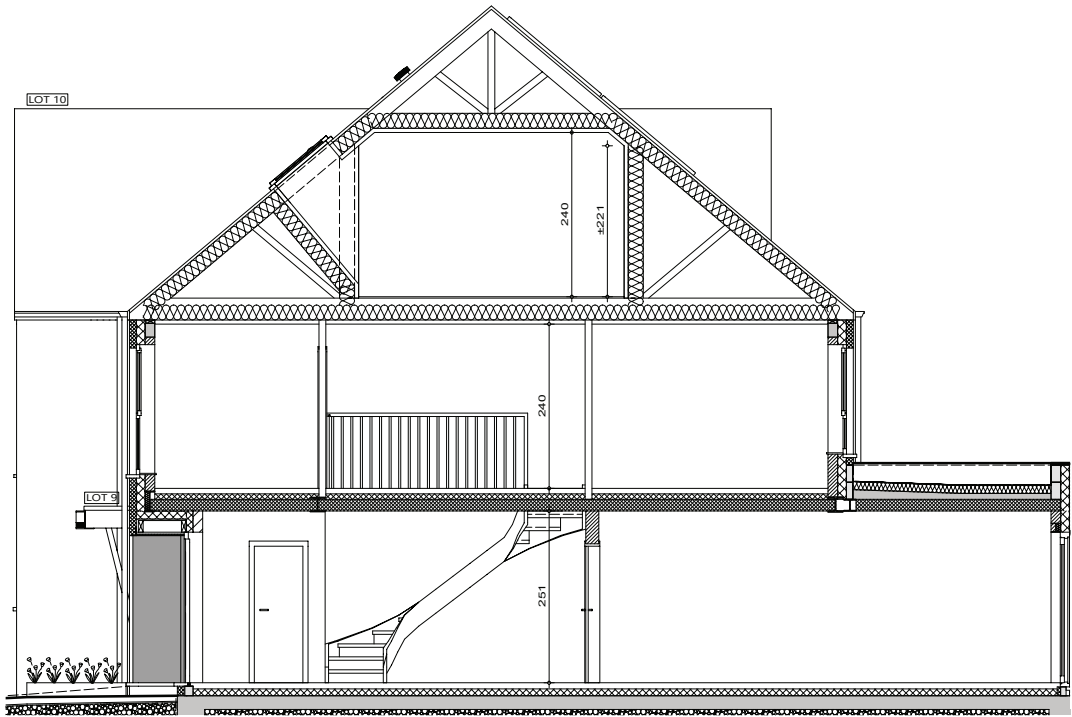
Coupe
