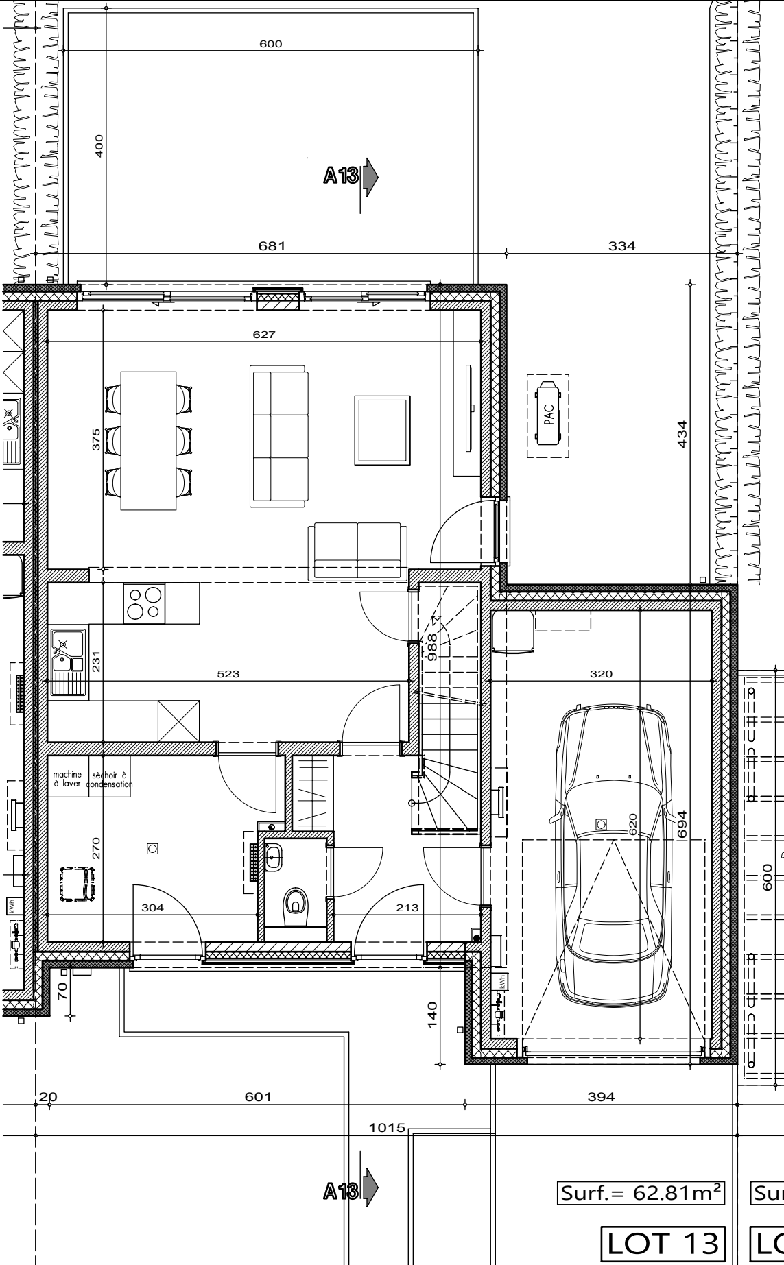
PLAN REZ-DE-CHAUSSEE
