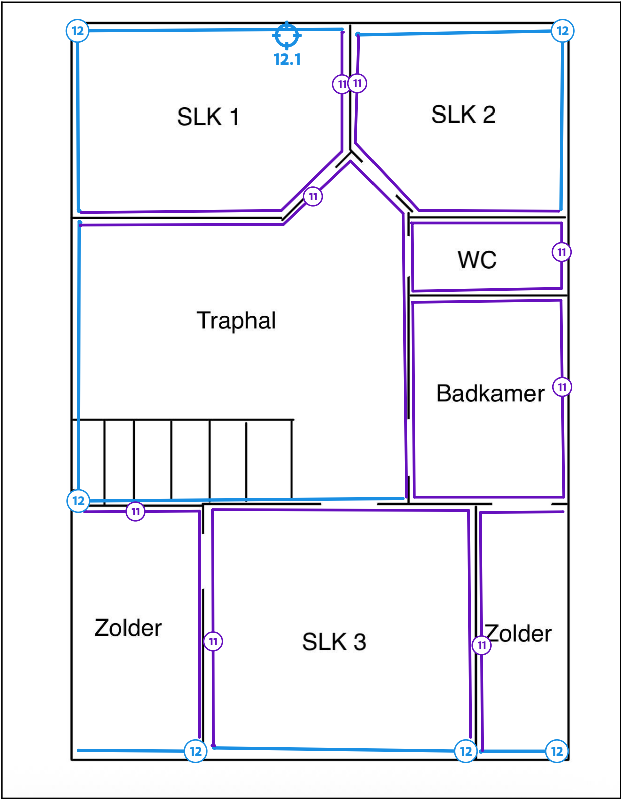
Legende van plan 1.4: Eerste verdiep
