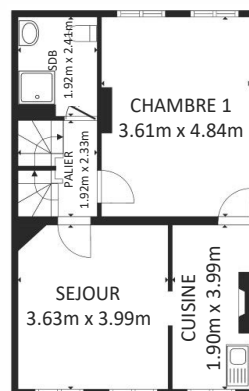
2ème ETAGE
