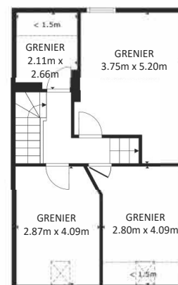
3ème ETAGE
